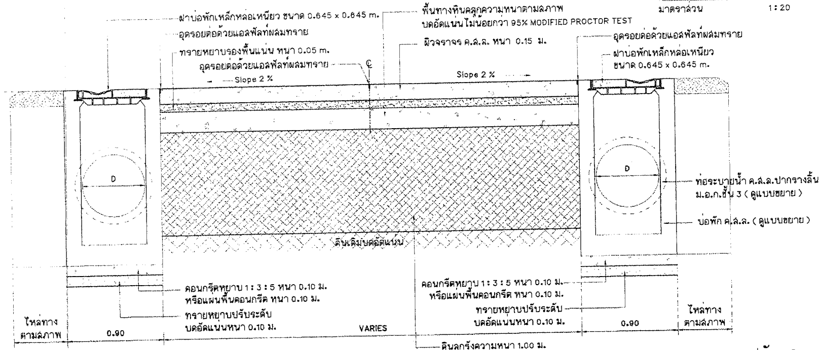
แบบขยายรูปตัด 2
