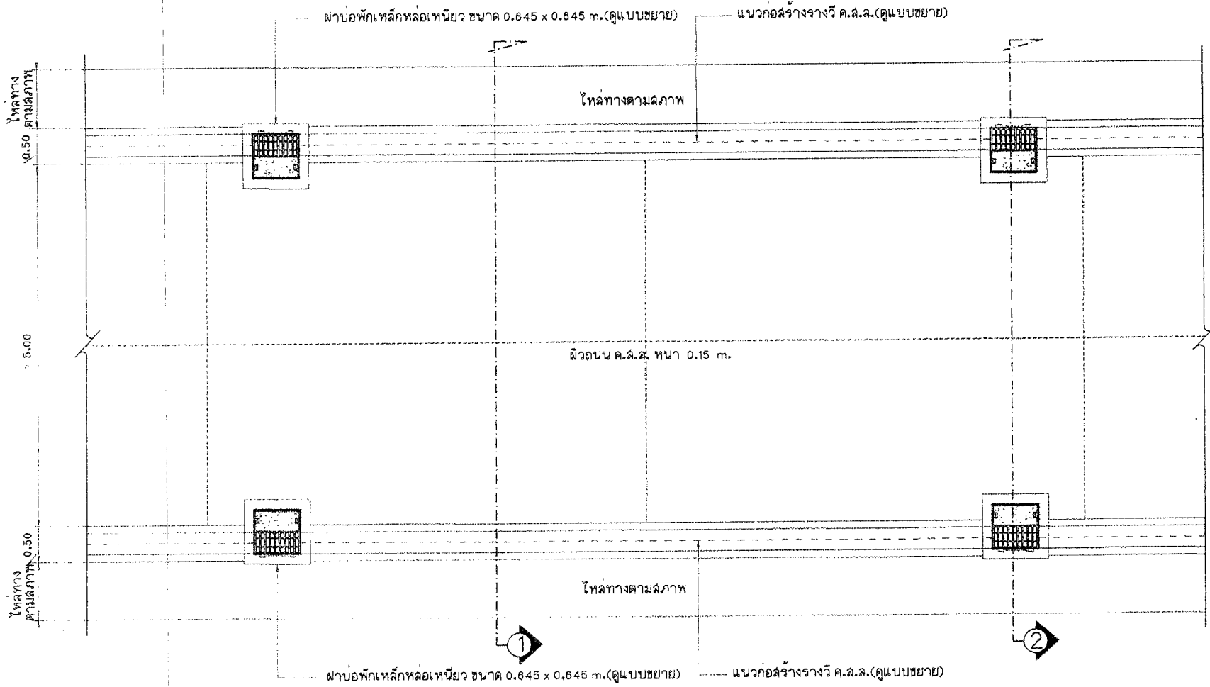
แปลนถนน และการวางบ่อพัก คสล. มาตรฐาน 1 : 50
