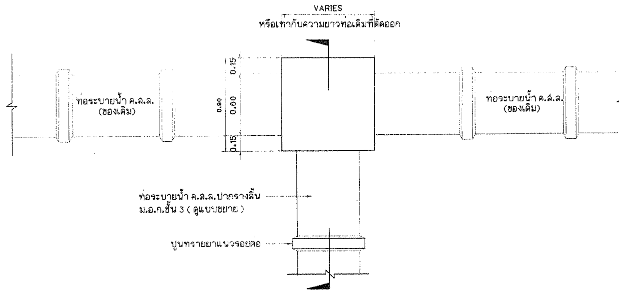
แบบการเชื่อมต่อในกรณีเชื่อมกับท่อระบายน้ำของเดิม มาตราส่วน 1:20
