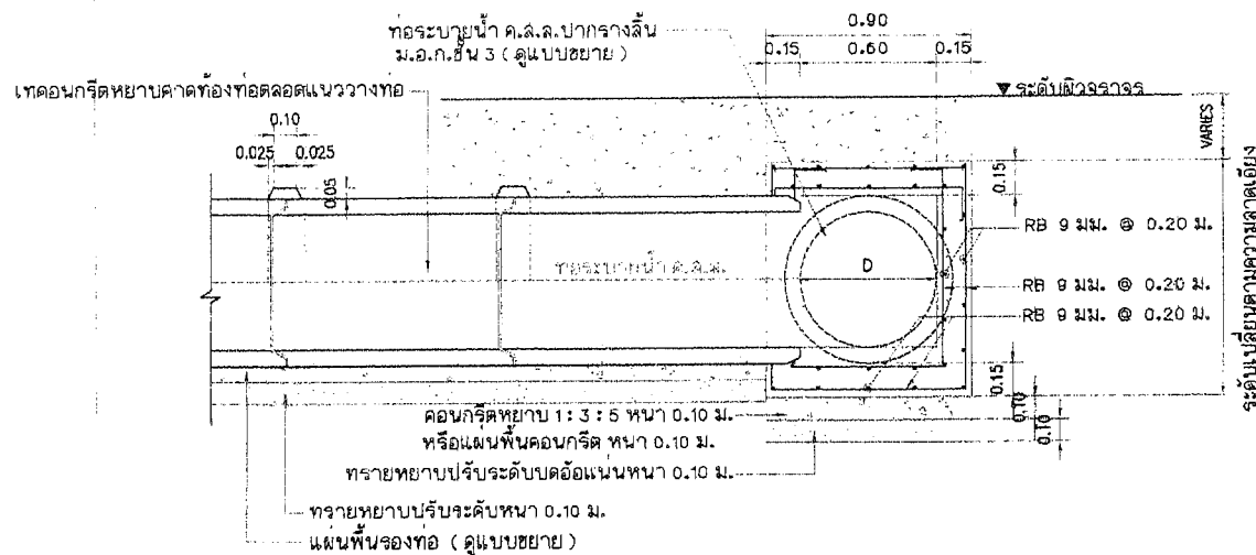
รูปตัดการเชื่อมต่อในกรณีเชื่อมกับท่อระบายน้ำของเดิม มาตราส่วน 1:20
