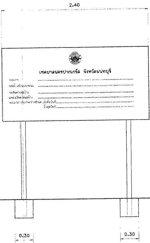
รูปด้านหน้าป้ายโครงการ มาตราส่วน 1:25
