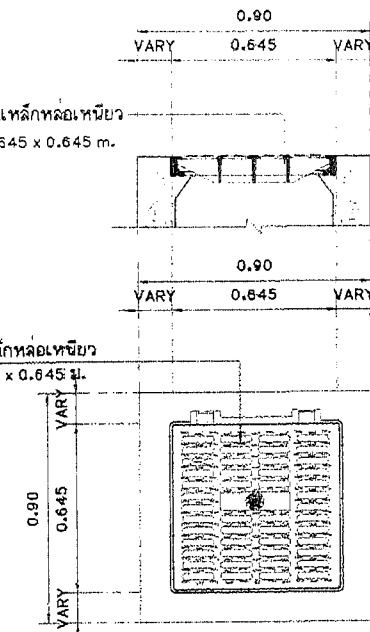
แบบขยายฝาบ่อพักเหล็กหล่อเหนียว 2
