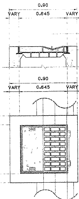
แบบขยายฝาบ่อพักเหล็กหล่อเหนียว 1
