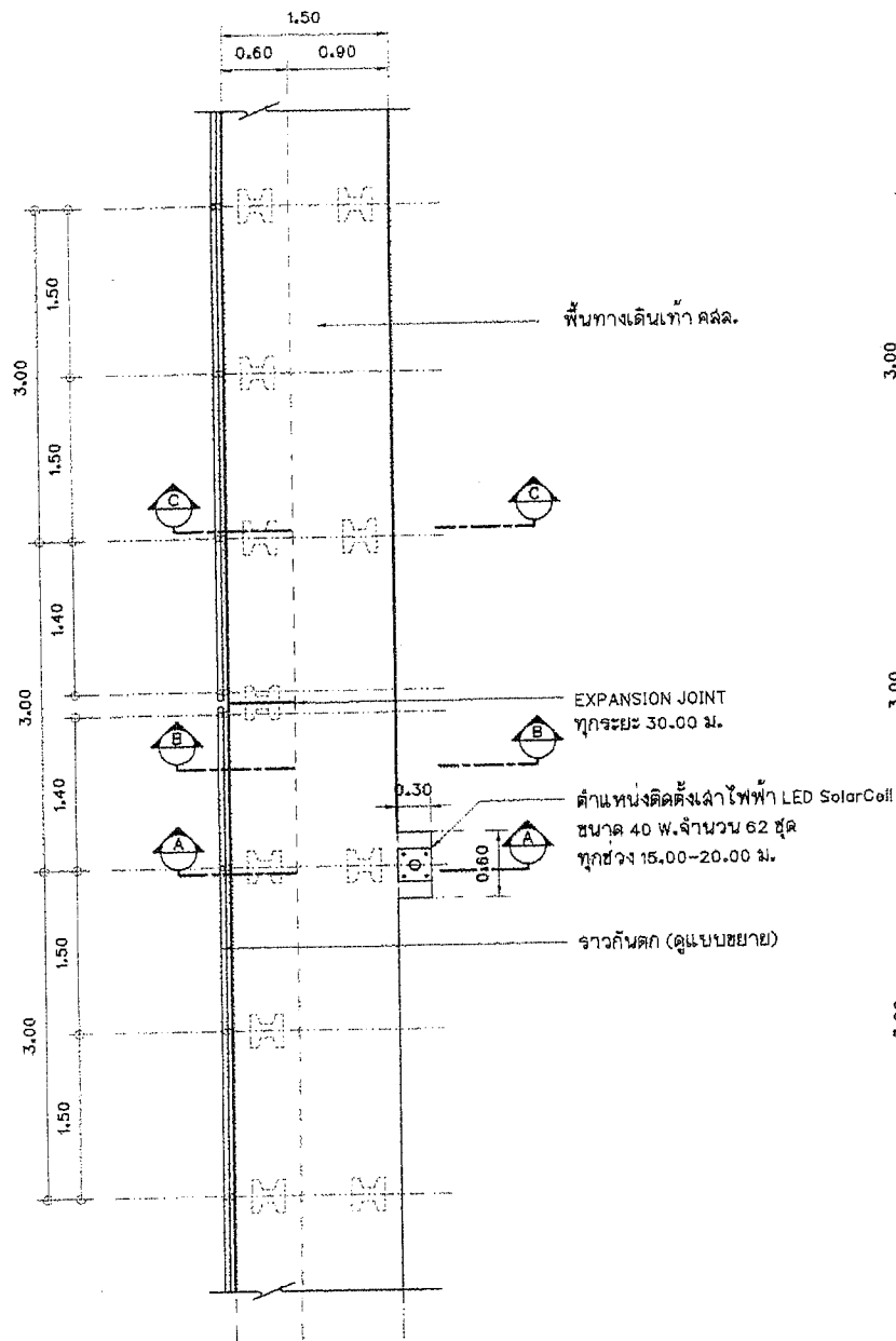
แปลนเขื่อน คลล. มาตราส่วน 1:50
