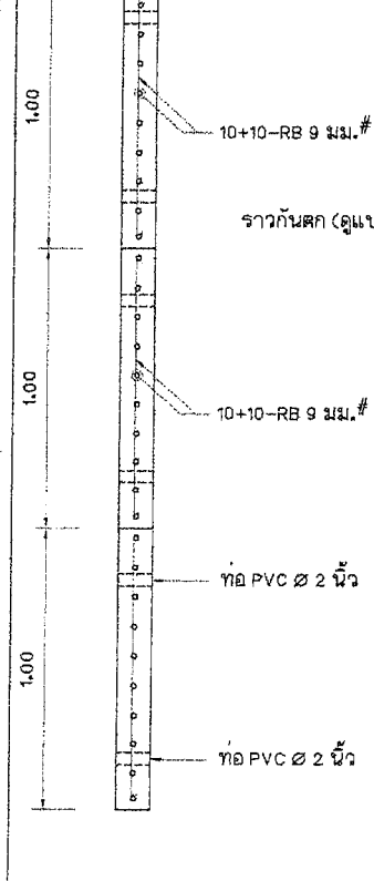
แบบขยายแผ่นกันดิน คลล์ มาตราส่วน 1:20
