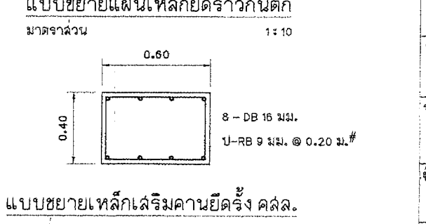
แบบขยายรูปตัดคานทับหลัง ค.ล.ล. มาตราส่วน 1:20
