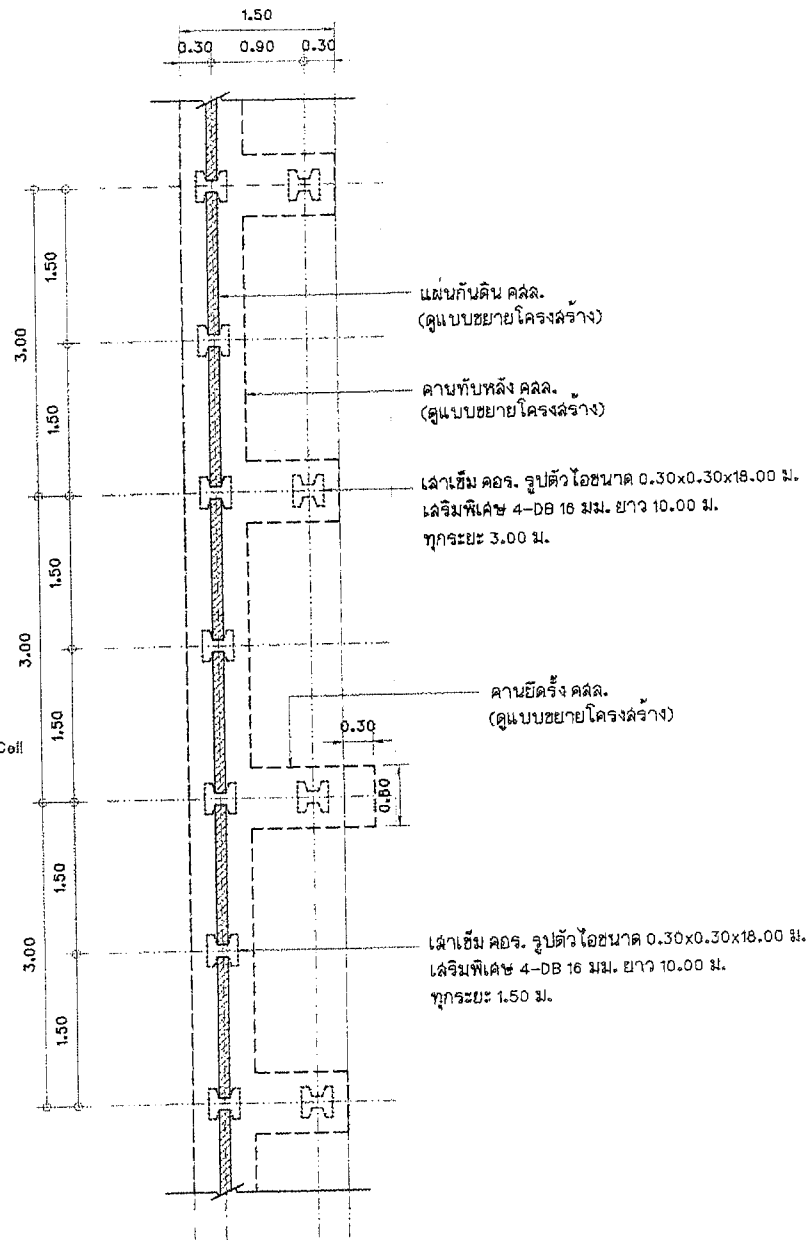
แปลนเสาเข็มแผ่นกำแพงกันดิน คลล., คาน คลล. มาตราส่วน 1:50
