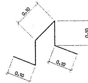
แบบขยายเหล็กขัดรับเหล็กตะแกรง NON TO SCALE
