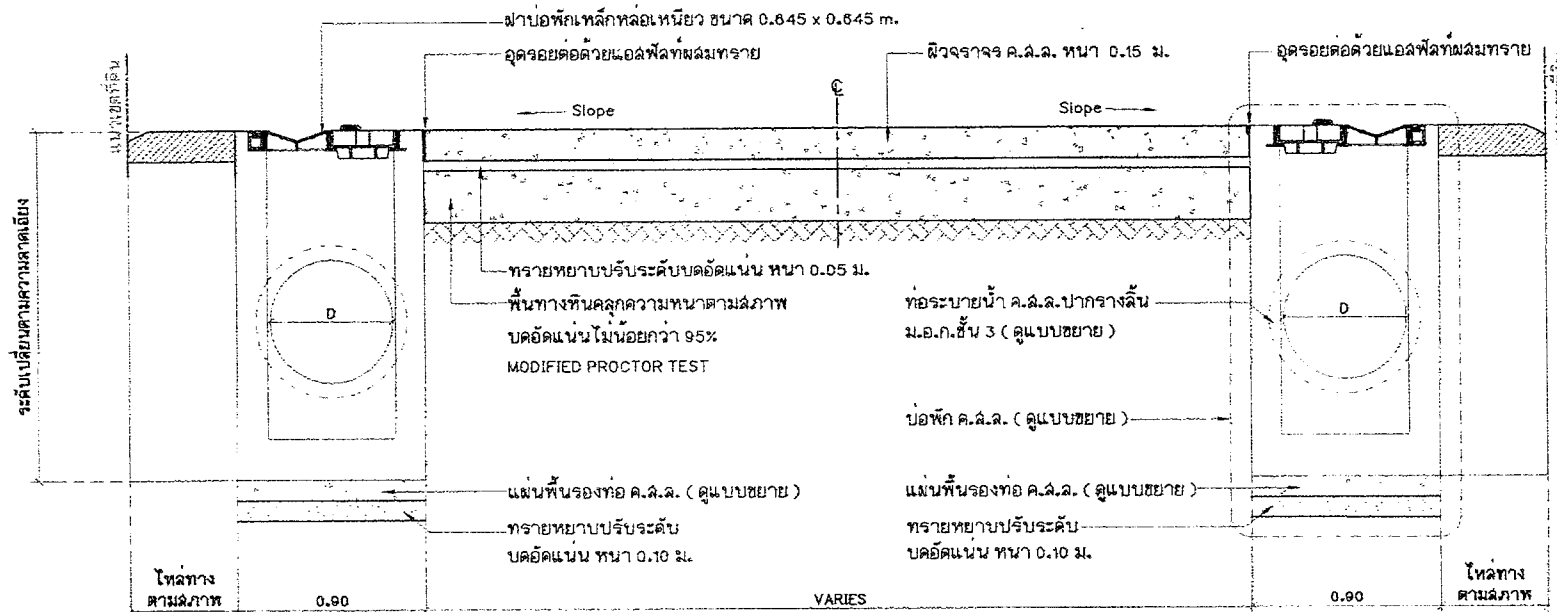
รูปตัด มาตราส่วน 1 : 25
