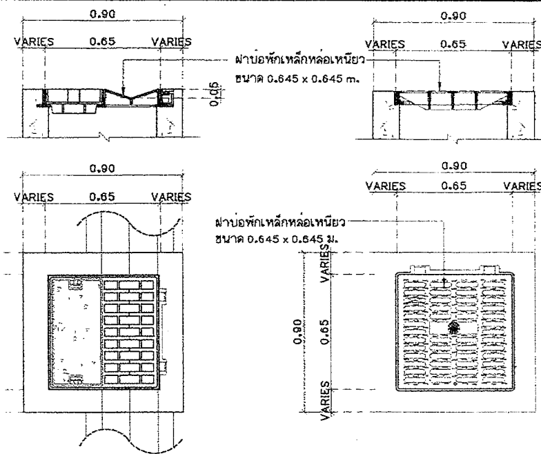
แบบขยายบ่อพักเหล็กหล่อเหนียว 1 มาตราส่วน 1:20
