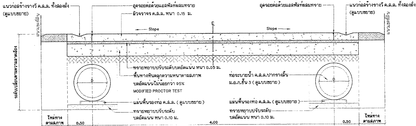
รูปตัด มาตราส่วน 1 : 25
