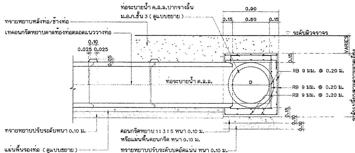
รูปตัด มาตราส่วน 1 : 25
