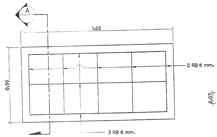
แบบขยายตัดขวางวิ คลล. มาตราส่วน 1 : 10
