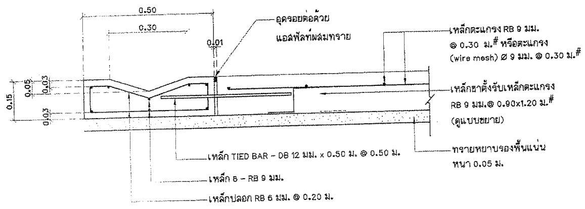
แบบขยายตัดขวางวิ คลล. มาตราส่วน 1 : 10
