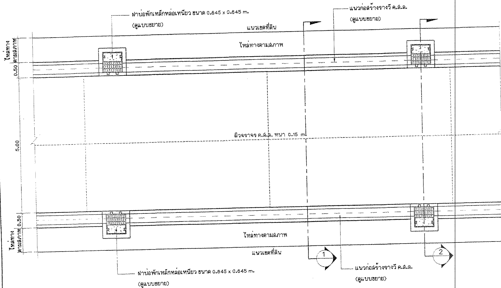
แปลนถนน และการวางบ่อพัก ค.ล.ล. มาตราส่วน 1 : 50
