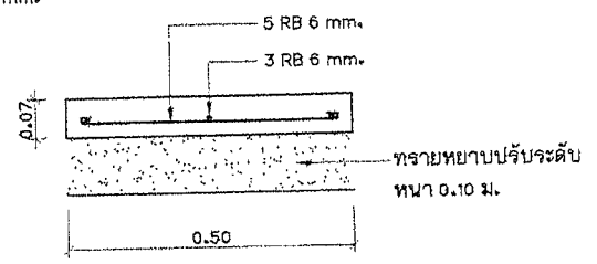
รูปตัด มาตราส่วน 1 : 10
