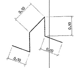
แบบขยายเหล็กขาตั้งรับเหล็กตะแกรง NON TO SCALE
