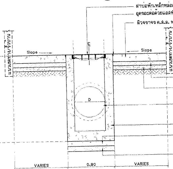
รูปตัด มาตราส่วน 1 : 25
