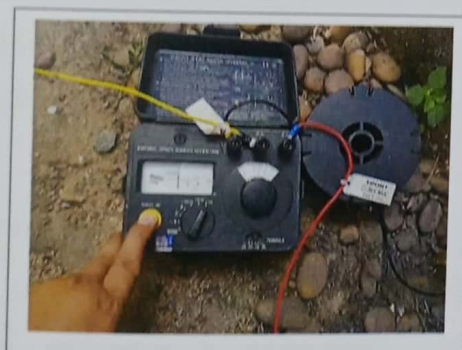
ลักษณะตัวนำไฟฟ้า และตัวนำต่อลงดิน
