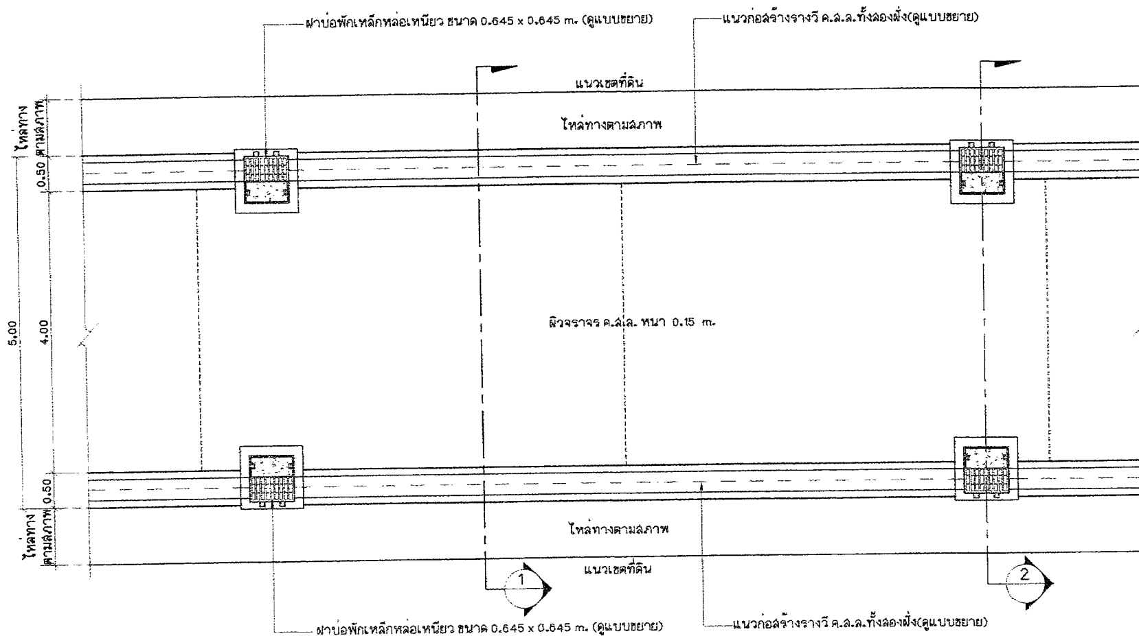
แปลนถนน และการวางบ่อพัก คสล. มาตราส่วน 1 : 50
