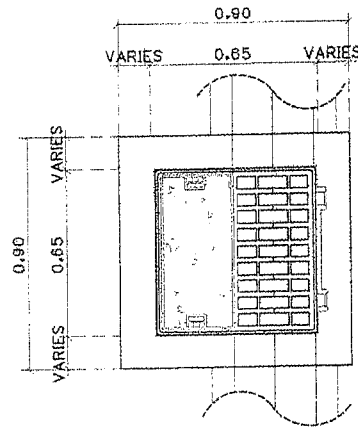
แบบขยายฝาบ่อพักหลักหลอเหนือ 1 มาตราส่วน 1:20
