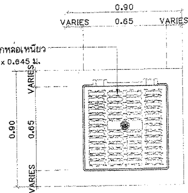
แบบขยายฝาบ่อพักหลักหลอเหนือ 2 มาตราส่วน 1:20
