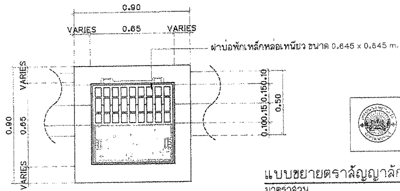
แบบขยายรางวัด มาตราส่วน 1:20
