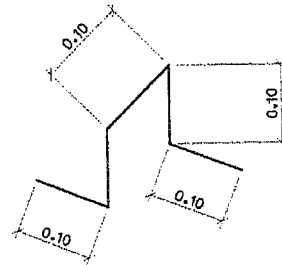
แบบขยายเหล็กรัดรับเหล็กตะแกรง NON TO SCALE
