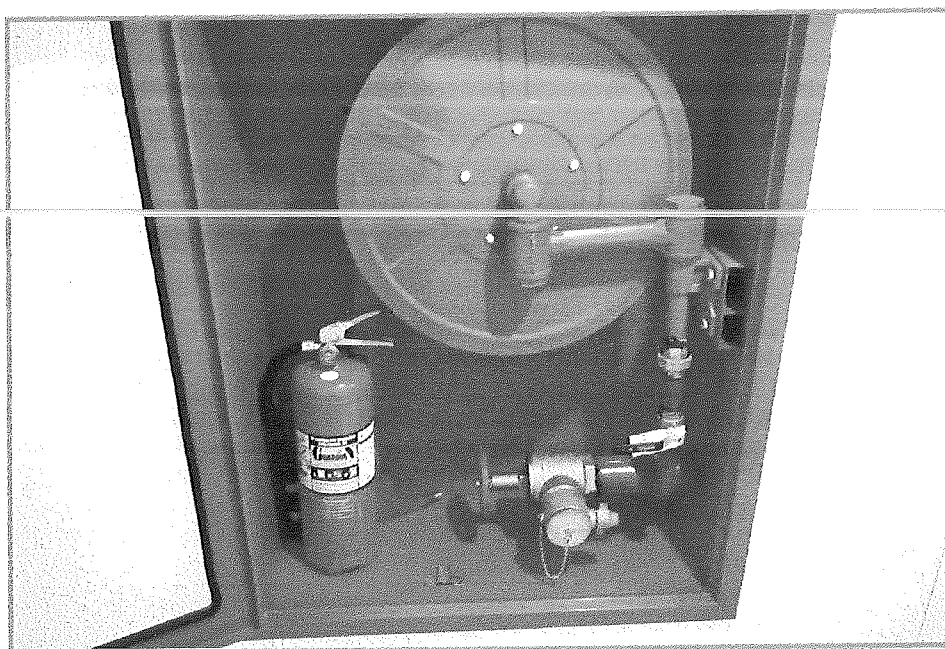
การติดตั้งถังดับเพลิงและตู้หัวฉีดน้ำดับเพลิง
