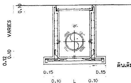
รูปตัดบ่อพัก คลล์.ลำเจ้าเจ็ฐ มาตราส่วน 1:25
