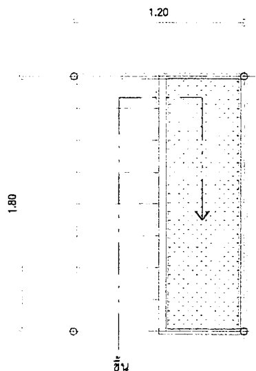
แปลนบันไดวงขึ้นดาดฟ้า มาตราส่วน 1:25
