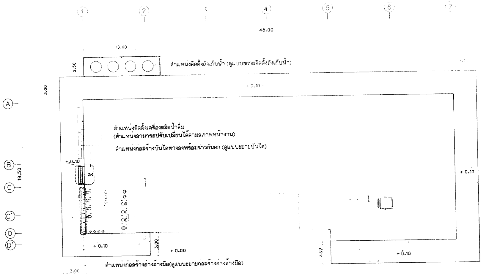
แปลนหลังปรับปรุงอาคาร 4 ชั้น 1 มาตราส่วน 1:200
