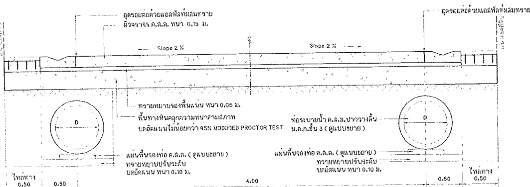
แบบขยายรูปตัด 1
