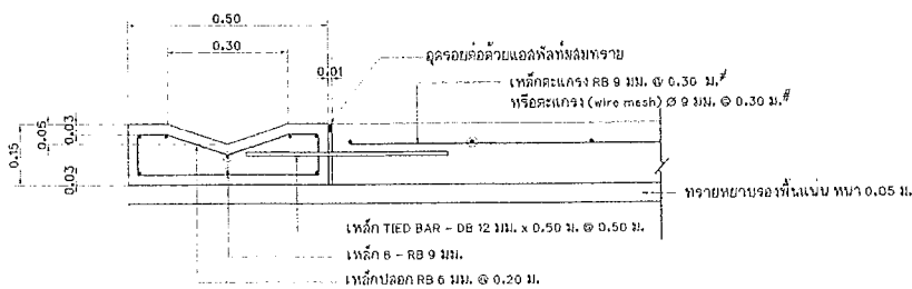
ขยายตัดขวางวิ. คลล. มาตราส่วน 1 : 10
