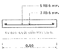
แบบขยายรูปตัดแผ่นพื้นรองท่อ มาตราส่วน 1 : 10
