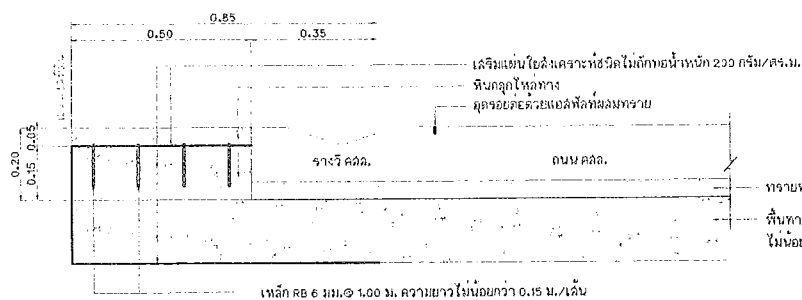
แบบขยายรูปตัดการติดตั้งแผ่นใยสังเคราะห์แผ่น มาตราส่วน 1 : 10
