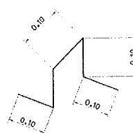
แบบขยายเหล็กขาตั้งรับเหล็กตะแกรง มาตราส่วนตามกำหนด
