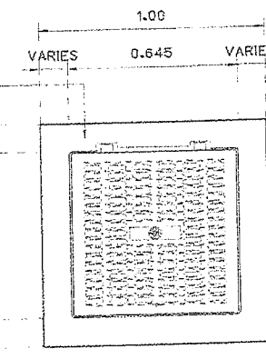
แบบขยายฝาบ่อพักเหล็กหล่อเหนียว 2 มาตราส่วน 1 : 25
