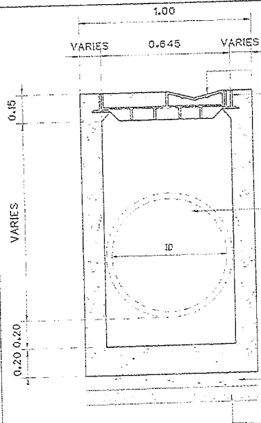
แบบขยายรูปตัด บ่อพัก คสล. มาตราส่วน 1 : 25
