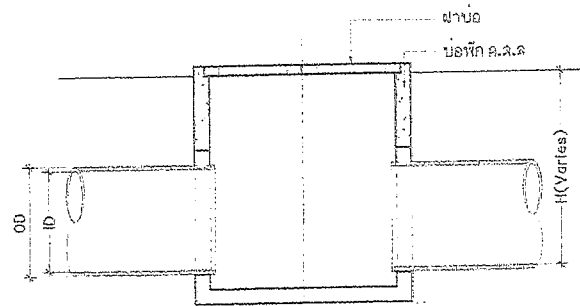
การประสานท่อ HDPE เข้าบ่อ ค.ส.ล.
