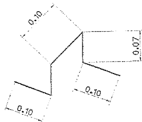
แบบขยายเหล็กขาตั้งรับเหล็กตะแกรง (ผิว คสล.หนา 0.12 ม.)
