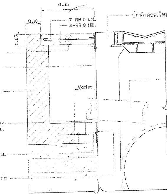
รูปตัด A มาตราส่วน 1:10
