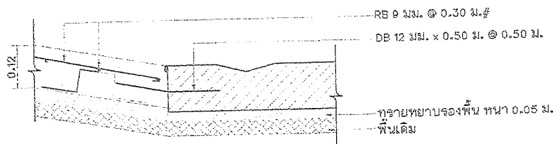
แบบขยายรูปตัด 3 (ทางเข้าบ้าน)
