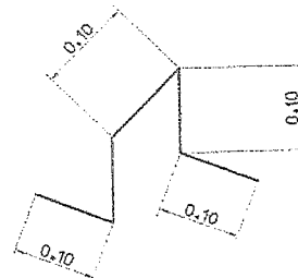
แบบขยายเหล็กขาตั้งรับเหล็กตะแกรง (ผิว คสล.หนา 0.15 ม.)
