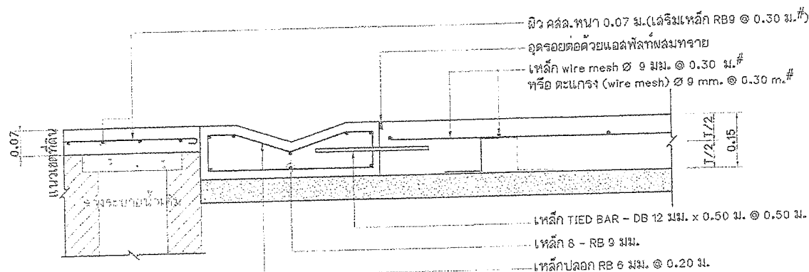
ขยายตัดขวางวี คสล.
