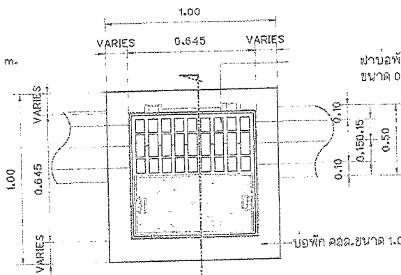
แบบขยายฝาบ่อพักเหล็กหล่อเหนียว 1 มาตราส่วน 1 : 25
