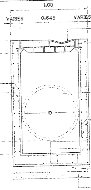
แบบขยายรูปตัดโครงสร้าง บ่อพัก คสล. มาตราส่วน 1 : 25
