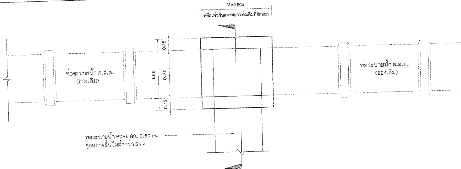
แผนการเชื่อมต่อในกรณีเชื่อมกับท่อระบายน้ำของเดิม มาตราส่วน 1:20
