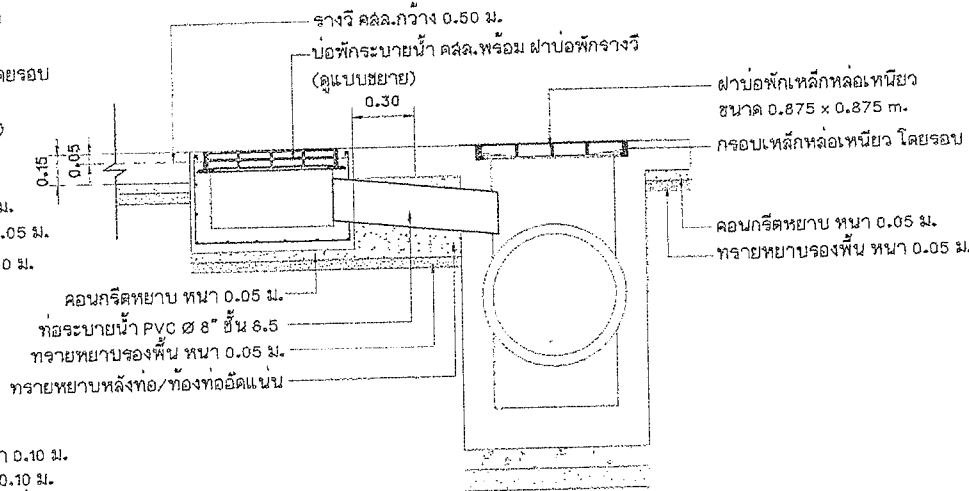
แบบขยายรูปตัดการเชื่อมต่อท่อ บ่อพัก(หัวมุม) มาตราส่วน 1:25
