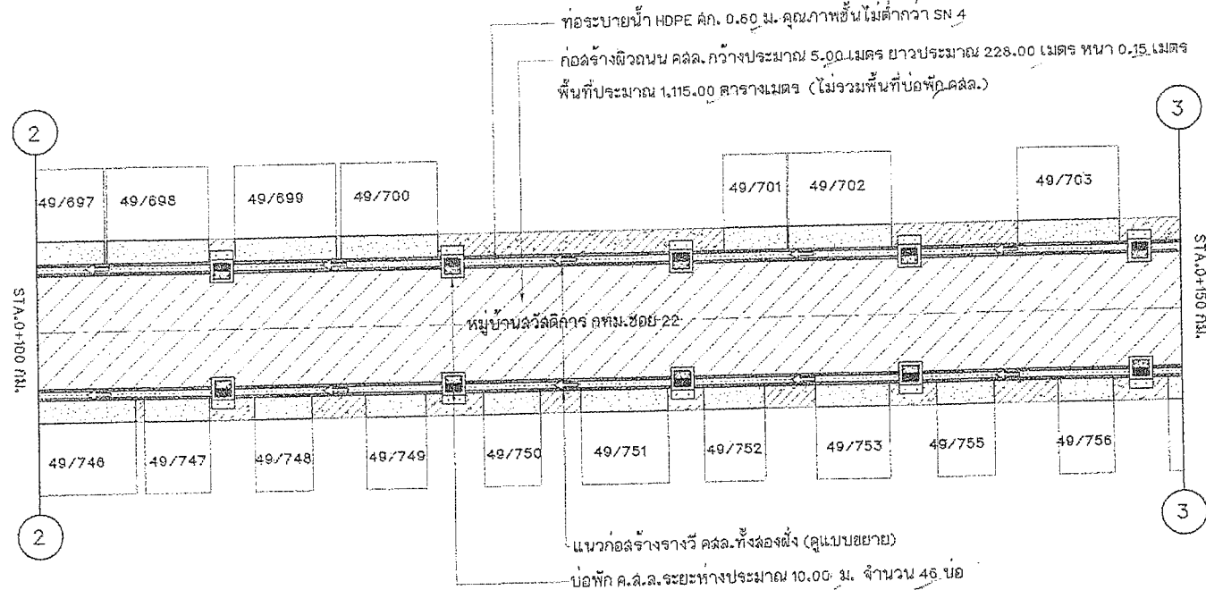
แปลนก่อสร้างปรับปรุงถนน และวางท่อระบายน้ำ มาตราส่วน 1 : 200
