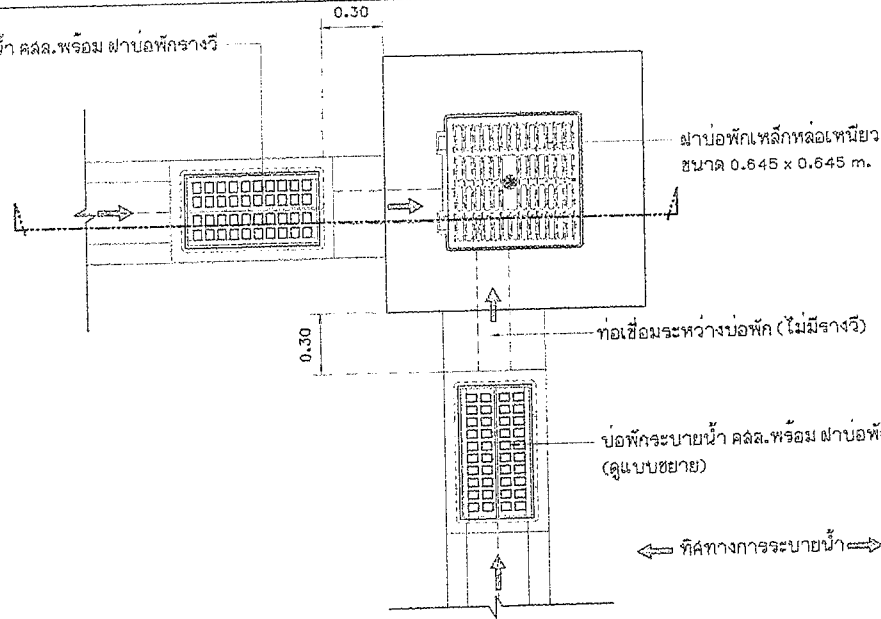
แปลนขยายช่องเปิดรับน้ำบ่อพัก(หัวมุม) มาตราส่วน 1:25
