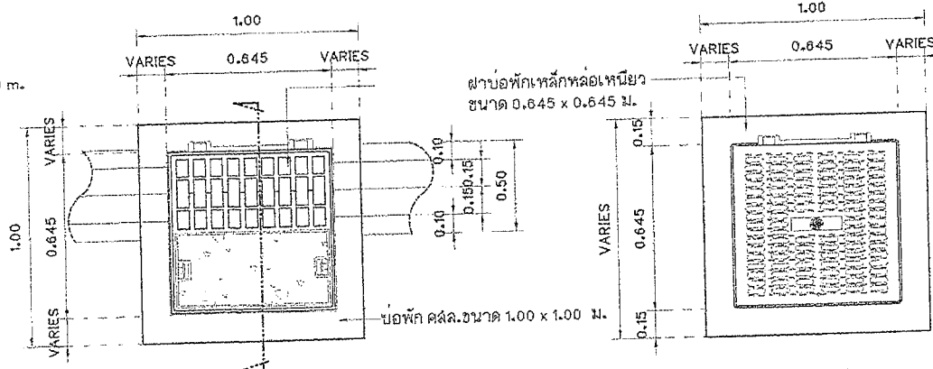
แบบขยายฝาครอบเหล็กหล่อเหนียว 2
