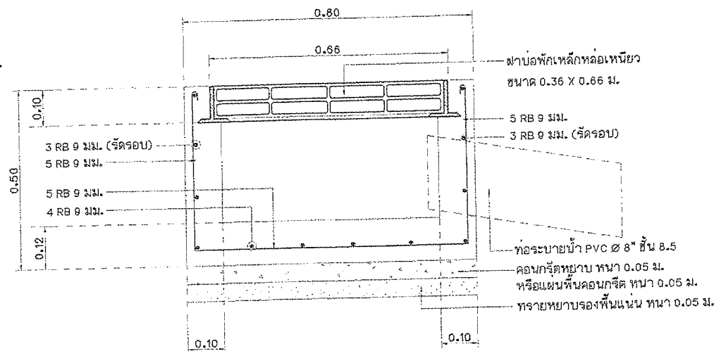
แบบขยายรูปตัด ② บ่อพักระบายน้ำ คลส. พร้อม ฝาบ่อพักรางวี มาตราส่วน 1 : 10
