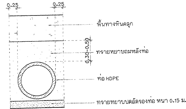
รูปตัดการวางท่อระบายน้ำ HDPE
