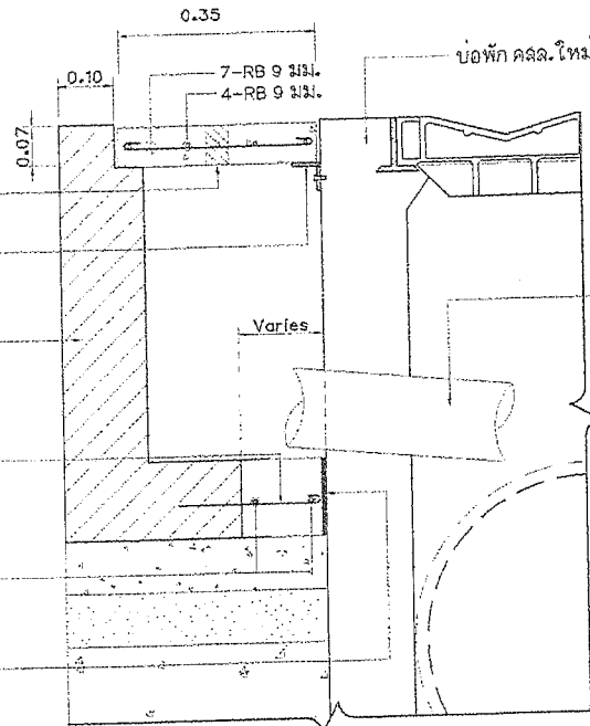
รูปตัด A มาตราส่วน 1:10
