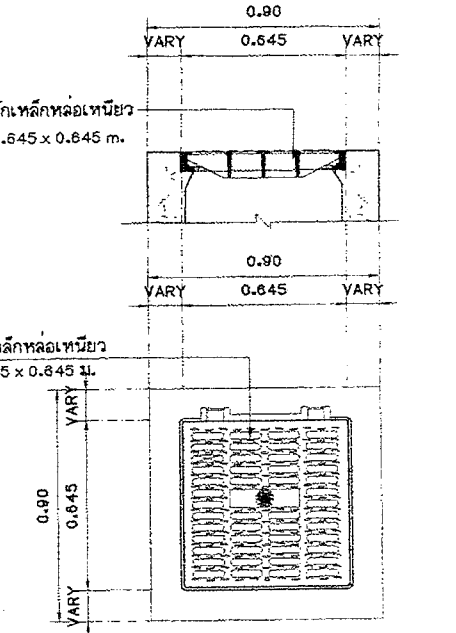
แบบขยายฝาบ่อพักเหล็กหล่อเหลี่ยม 2
