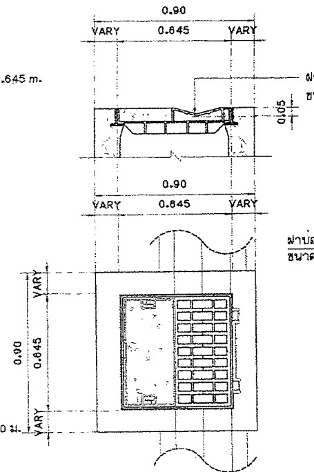
แบบขยายฝาบ่อพักเหล็กหล่อเหลี่ยม 1
