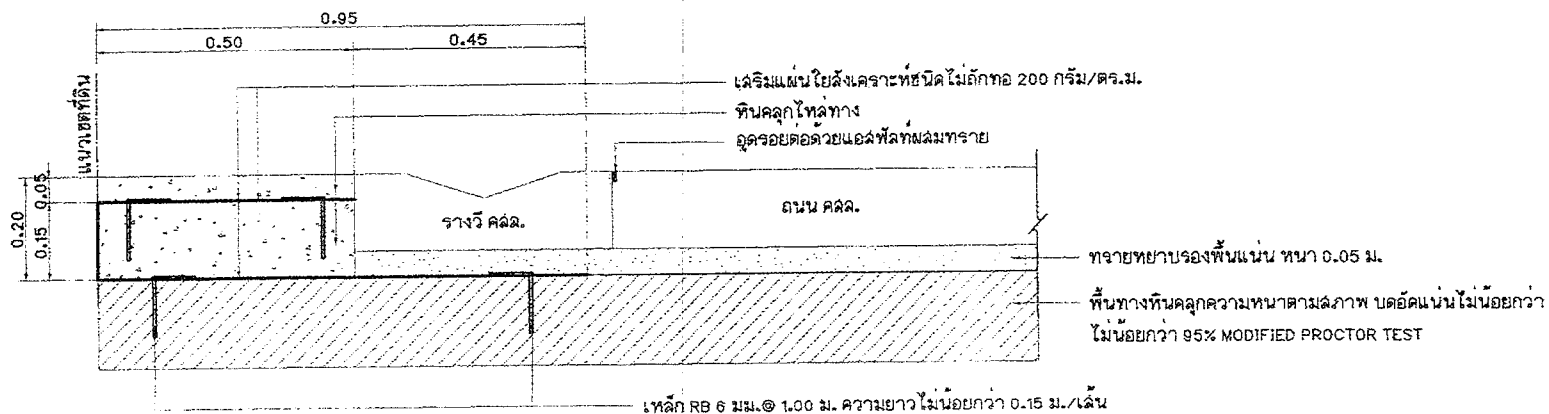
แบบขยายรูปตัดการติดตั้งแผ่นใยสังเคราะห์ที่แผ่น มาตราส่วน 1 : 10
