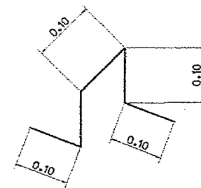
แบบขยายเหล็กขาตั้งรับเหล็กตะแกรง มาตราส่วนตามกำหนด
