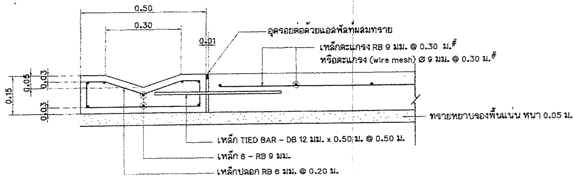
ขยายตัดขวางวิ คสล. มาตราส่วน 1 : 10
