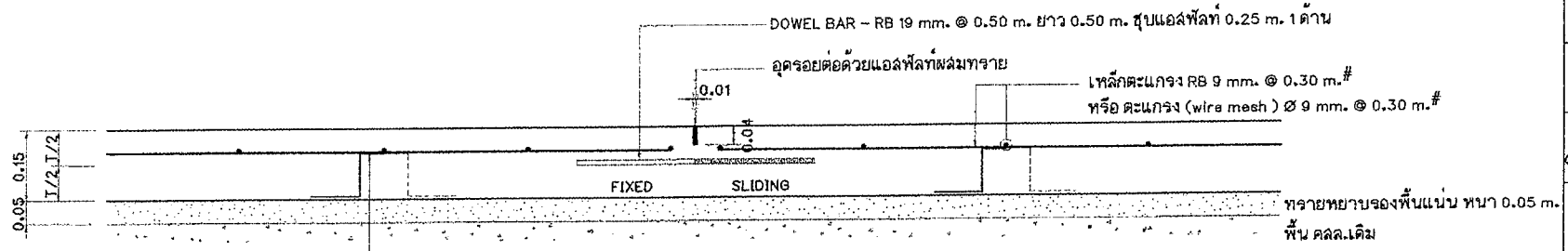
แบบขยาย TRANSVERSE JOINT มาตราส่วน 1:10 ทุกระยะ 6.00 m.
