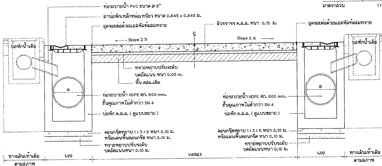
แบบขยายรูปตัด 2 มาตราส่วน 1:20
