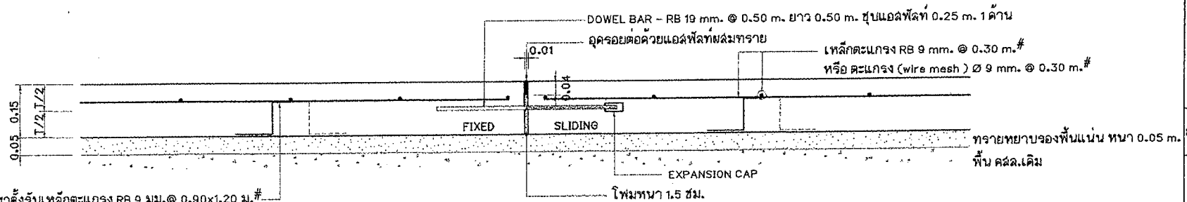
แบบขยาย EXPANSION JOINT มาตราส่วน 1:10 ทุกระยะ 30.00 m.
