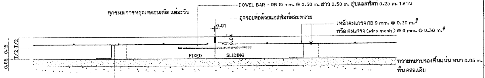
แบบขยาย CONSTRUCTION JOINT มาตราส่วน 1:10
