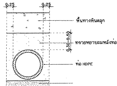
ท่อระบายน้ำ HDPE
