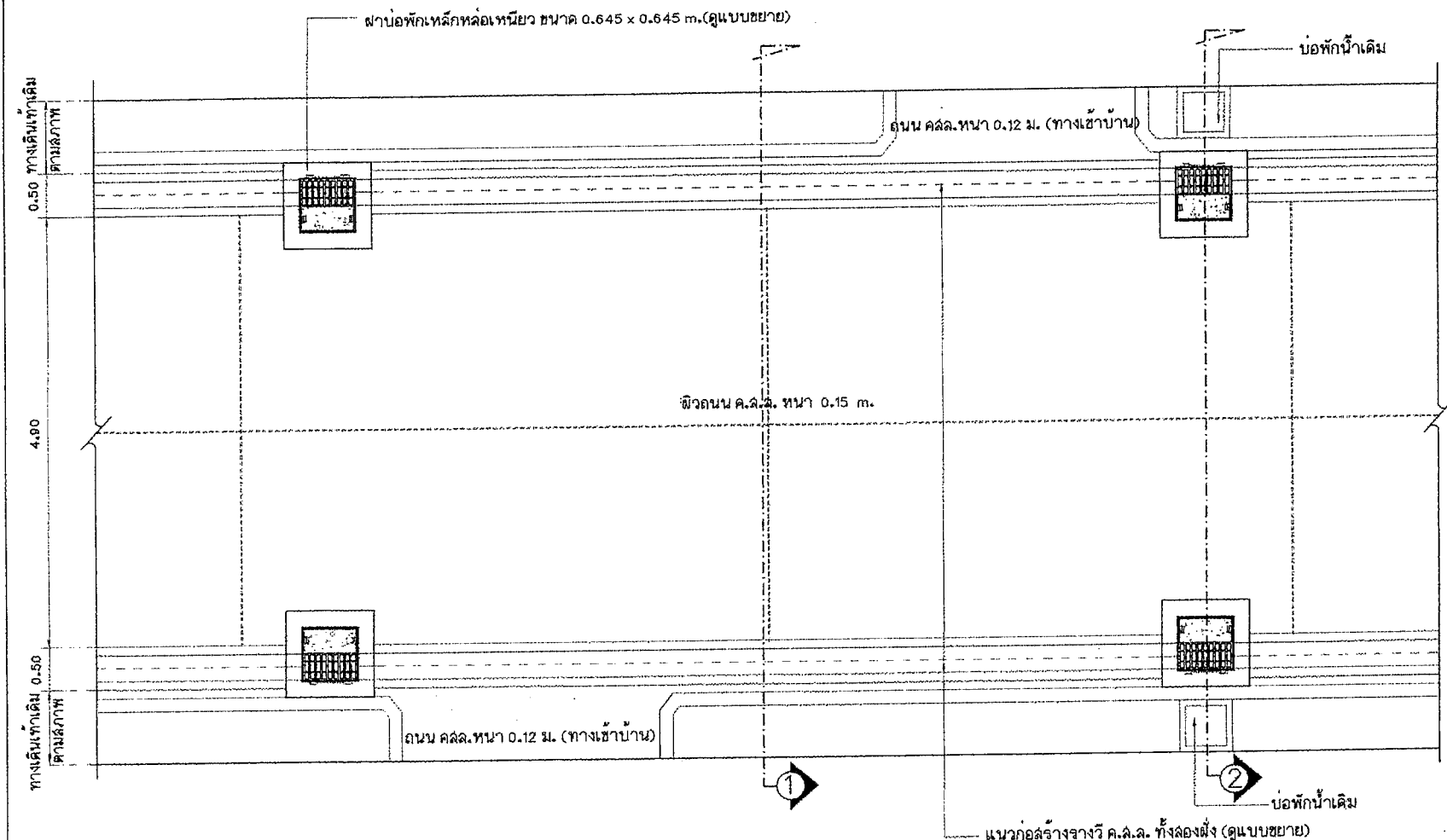
แปลนถนน การวางบ่อพัก คสล. และทางเข้าบ้าน มาตราส่วน 1 : 50
