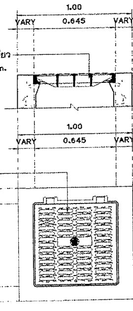
แบบขยายฝาบ่อพักเหล็กหล่อเหนียว 2 มาตราส่วน 1:20
