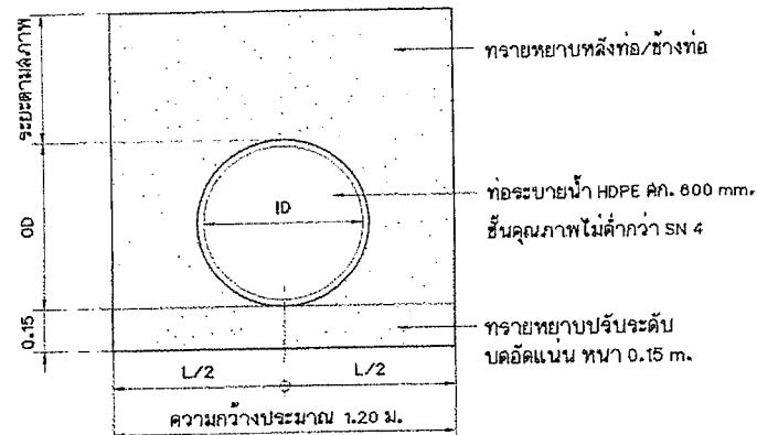
แบบขยายการวางท่อระบายน้ำ คสล. มาตราส่วน 1:20
