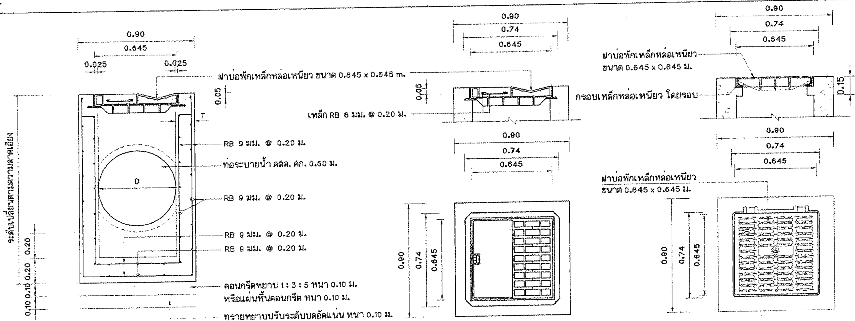
แบบขยายฝาบ่อพักเหล็กหล่อเหลี่ยม 2 มาตราส่วน 1:20
