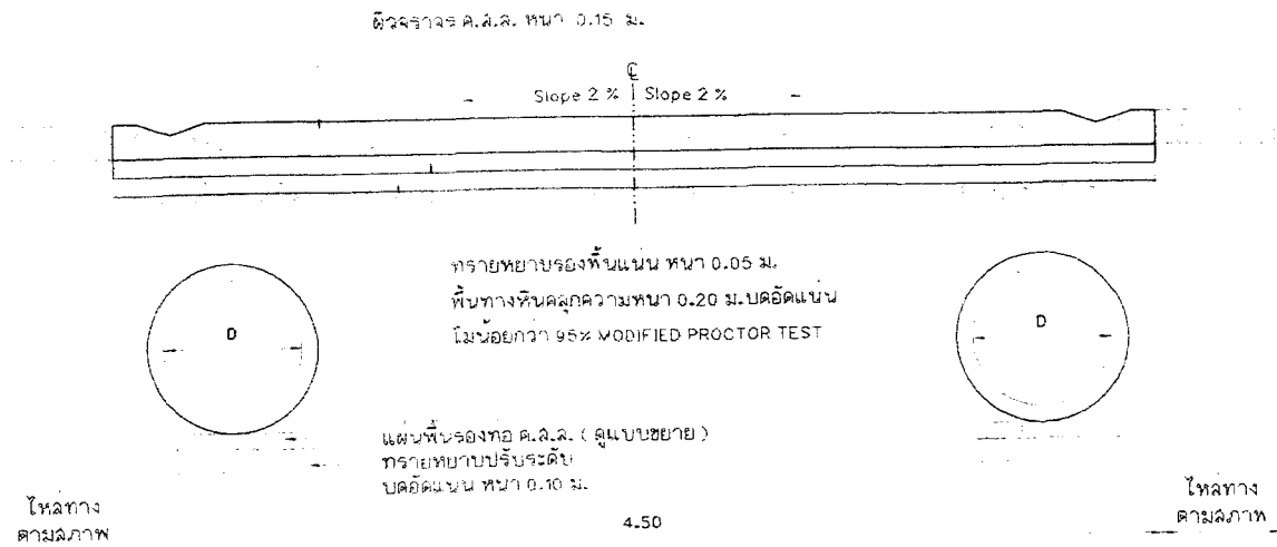
แบบขยายรูปตัด 1 (ช่วงความกว้าง 4.50 เมตร) มาตราส่วน 1:25
