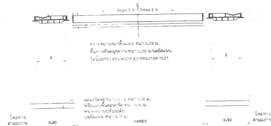
แบบขยายรูปตัด 2 (ช่วงความกว้าง 4.50 เมตร) มาตราส่วน 1:25
