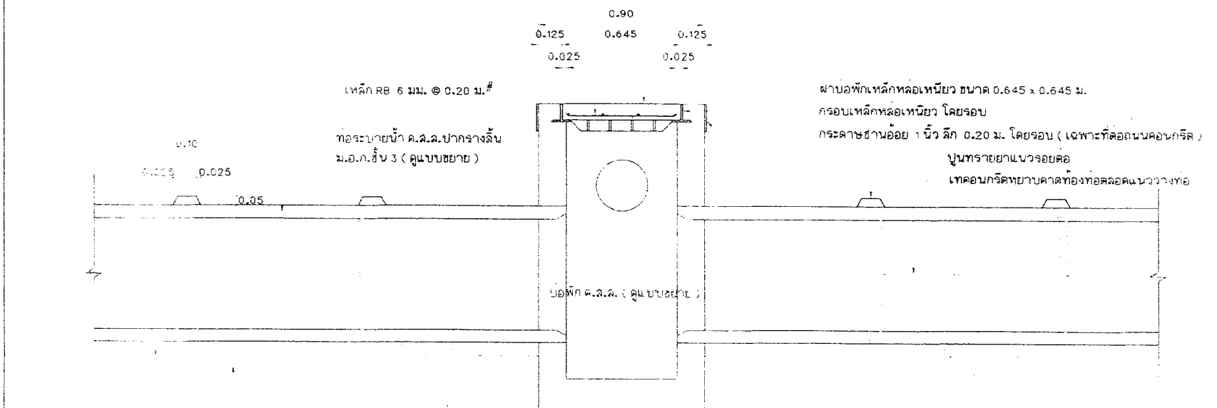
แปลนการวางทอระบายน้ำ มาตราส่วน 1:20
