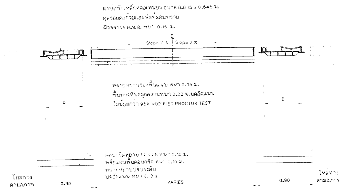
แบบขยายรูปตัด 2 (ช่วงความกว้าง 4.50 เมตร) มาตราส่วน 1:25
