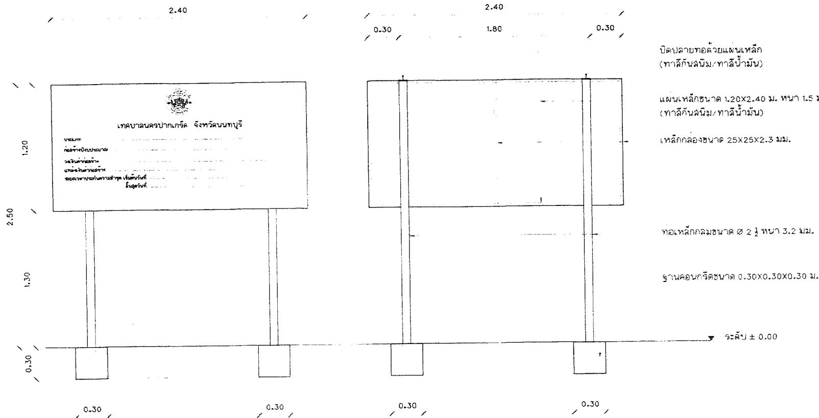
แบบป้ายโครงการ มาตรฐาน 1:25
