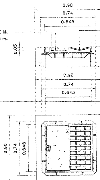
แบบขยายฝาครอบเหล็กหล่อเหนียว 1 มาตราส่วน 1:20
