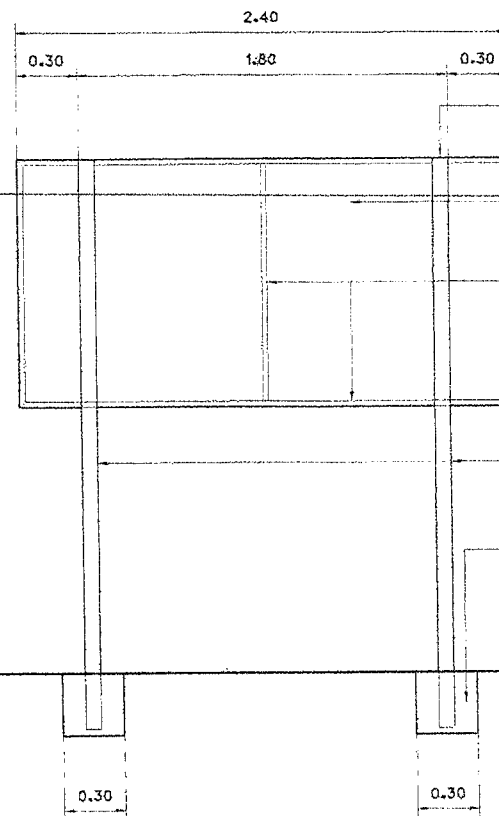
รูปด้านหลังป้ายโครงการ มาตราส่วน 1:25
