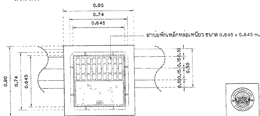
แบบขยายฝาครอบเหล็กหล่อเหนียว 1 มาตราส่วน 1:20
