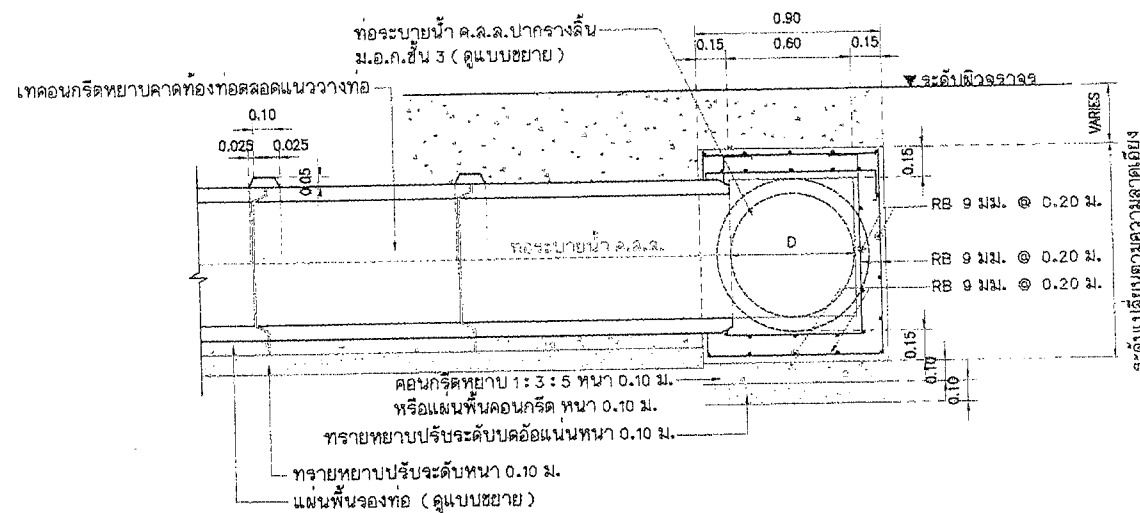
รูปตัดการเชื่อมต่อในกรณีเชื่อมกับท่อนบายน้ำของเดิม มาตราส่วน 1:20
