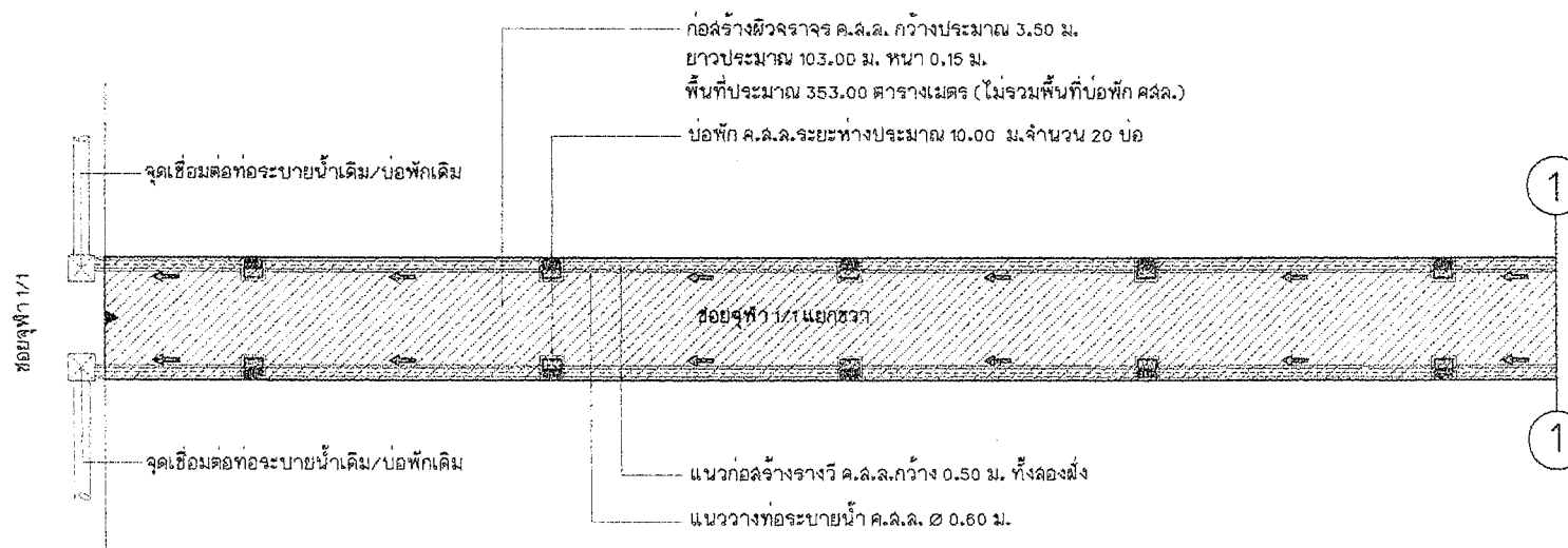
แปลนก่อสร้างถนน และท่อระบายน้ำ มาตราส่วน 1:200
