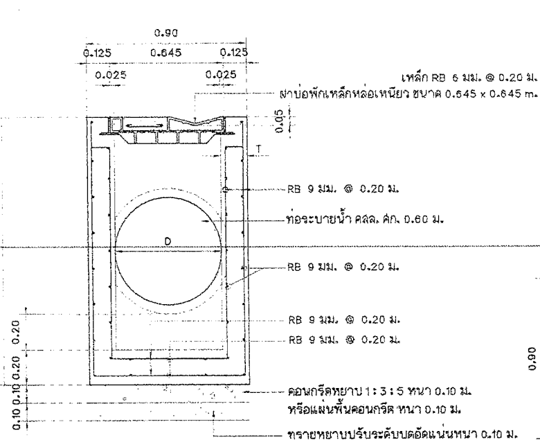
แบบขยายบ่อพัก ค.ส.ล. มาตรา ๑๖ 1:20
