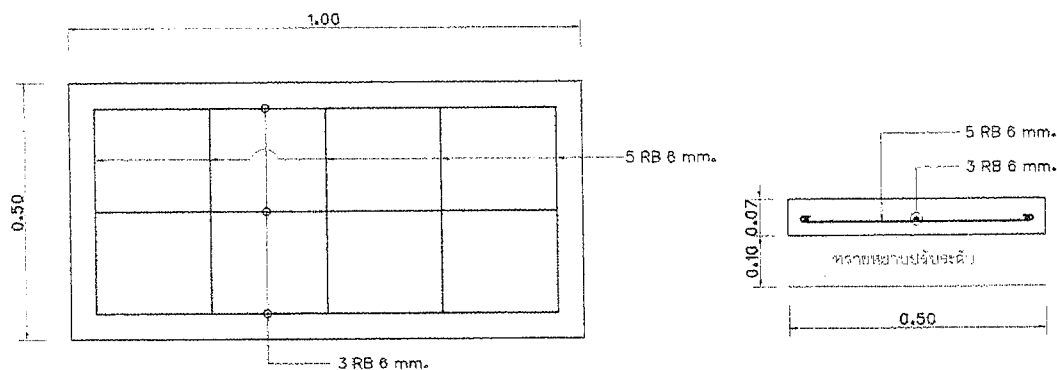
แบบขยายแผ่นพื้นรองท่อ มาตราส่วน 1 : 10
