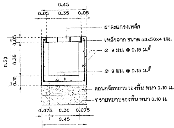
แบบขยายรูปตัดตรงระบายน้ำ คลล์. มาตราส่วน 1 : 15
