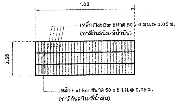
แบบขยายฝาดะแกรงเหล็ก มาตราส่วน 1 : 15
