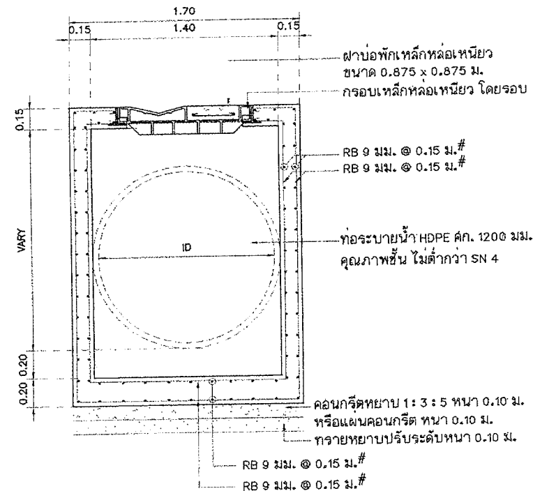
แบบขยายรูปตัด บ่อพัก คสล.
