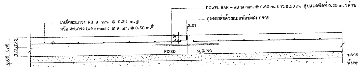
แบบขยาย EXPANSION JOINT ทุกระยะ 30.00 m. มาตราส่วน 1 : 10
