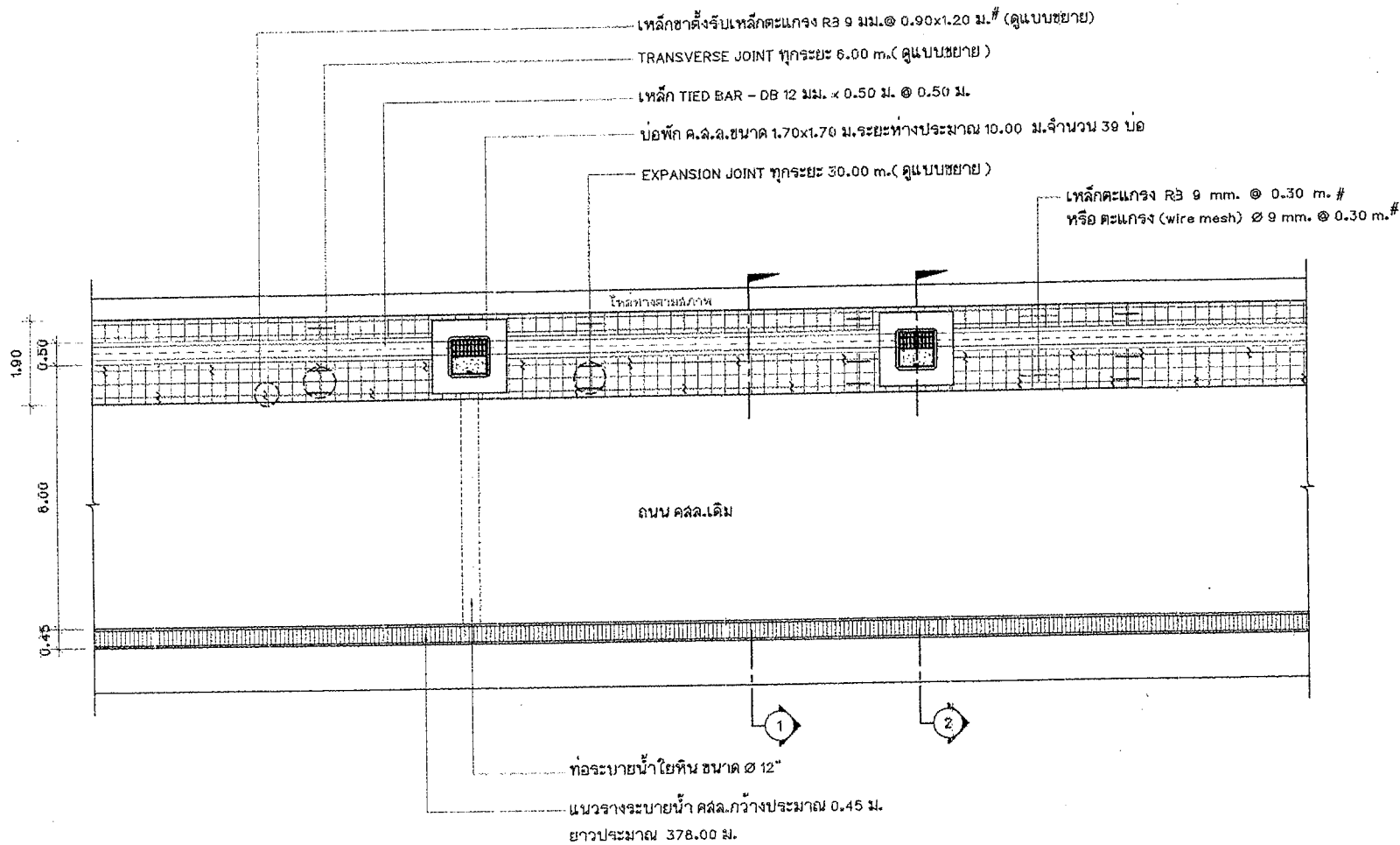
แปลนการวางเหล็กตะแกรงและรอยต่อถนน คสล. มาตราส่วน 1 : 100
