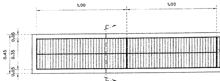
แบบขยายร่างระบายน้ำ คลล์. พร้อมฝาดะแกรงเหล็ก มาตราส่วน 1 : 15
