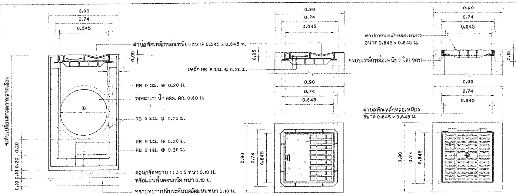
แบบขยายฝาบ่อพักเหล็กหล่อเหนียว 1 มาตราส่วน 1:20
