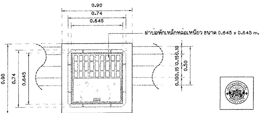
แบบขยายฝาบ่อพักเหล็กหล่อเหนียว 1 มาตราส่วน 1:20
