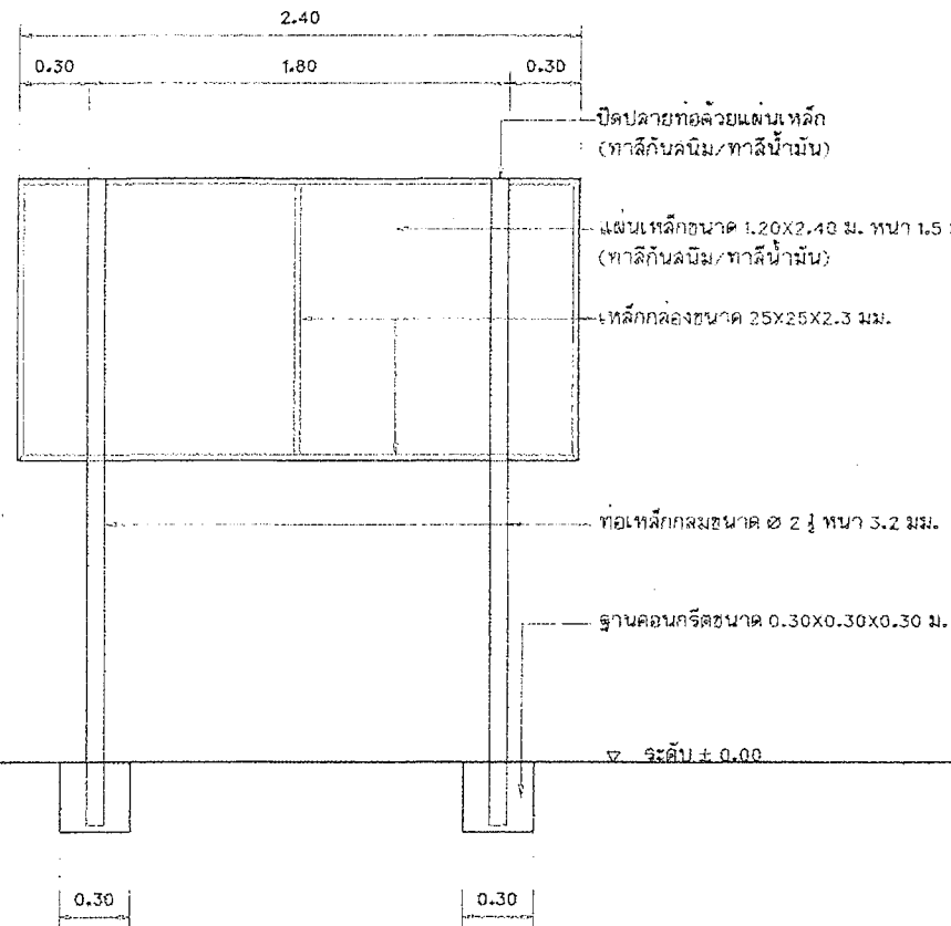
รูปด้านหลังป้ายโครงการ มาตราส่วน 1:25
