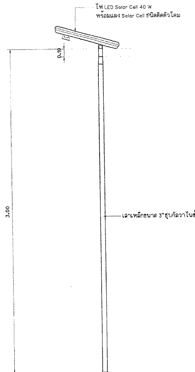
แบบขยายเสาไฟ มาตราส่วน 1:20
