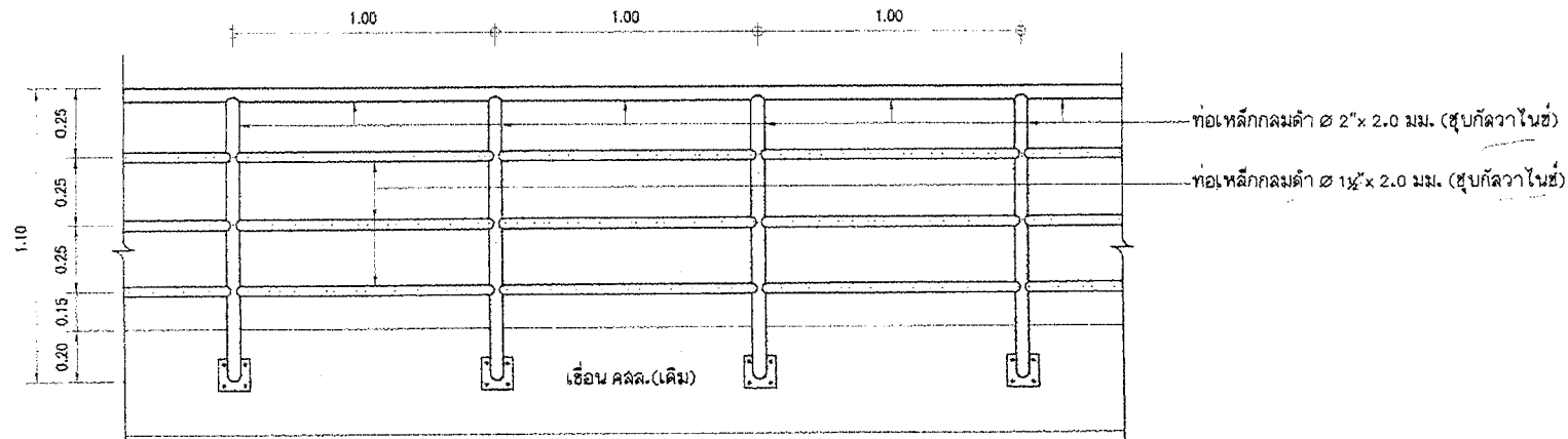
แบบขยาย รูปด้านหน้ารั้วเหล็กกันตก
