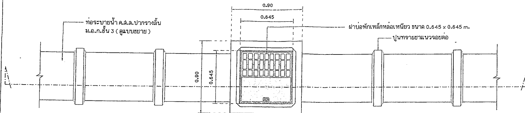
แปลนการวางท่อระบายน้ำ มาตราส่วน 1:20
