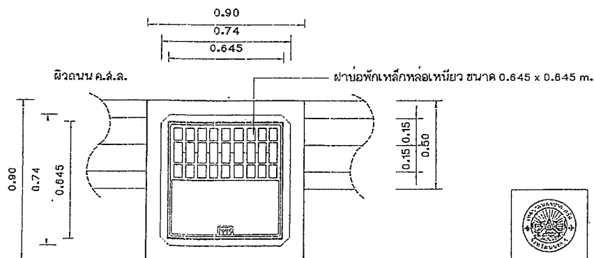
แบบขยายผ่าบอพักเหล็กหล่อเหนียว 1 มาตราส่วน 1:20
