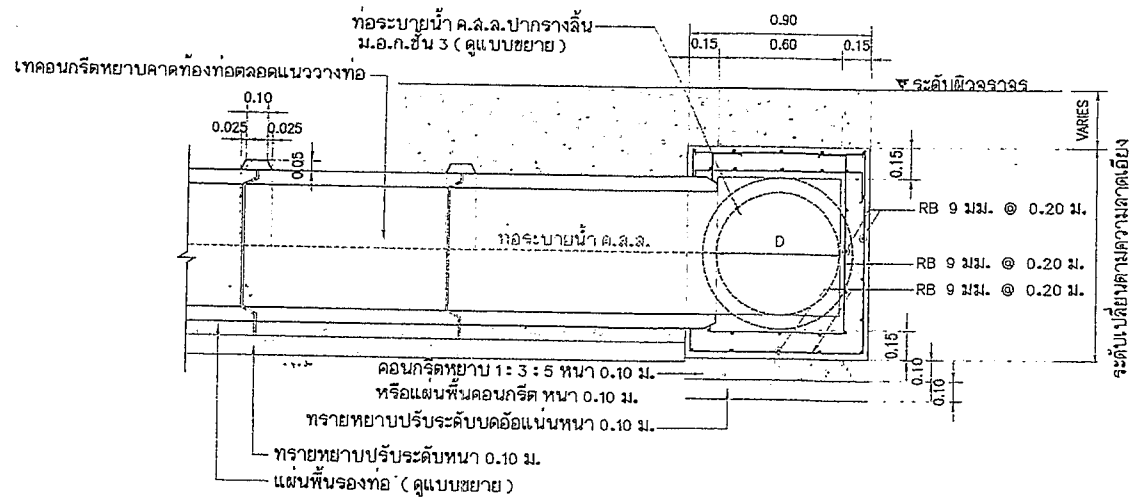
รูปตัดการเชื่อมต่อในกรณีเชื่อมกับทอระบายน้ำของเดิม
