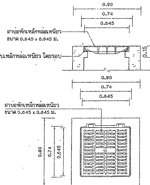
แบบขยายผ่าบอพักเหล็กหล่อเหนียว 2 มาตราส่วน 1:20
