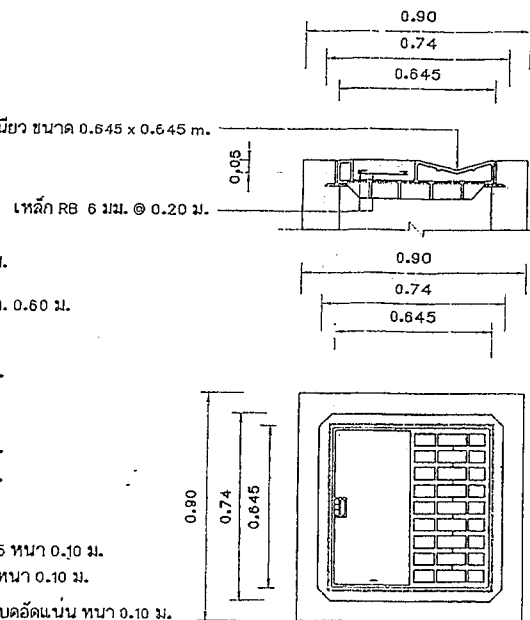
แบบขยายผ่าบอพักเหล็กหล่อเหนียว 1 มาตราส่วน 1:20
