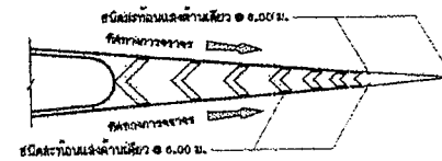
การติดตั้งปูมะทอนแสงเกาะกลางกรณีเดินรถทางเดียว
