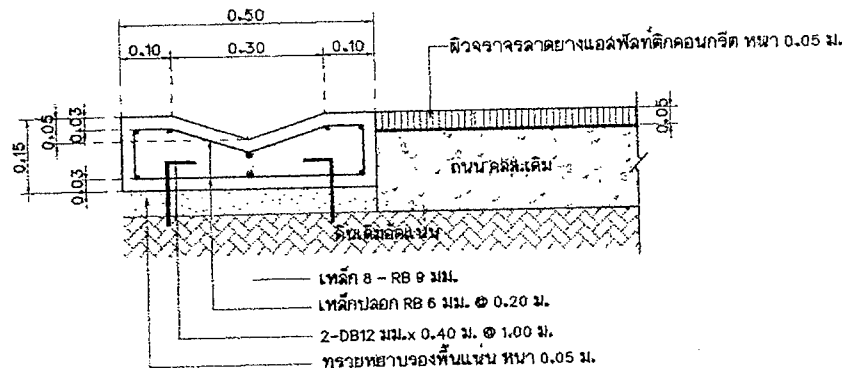
ขยายตัดขวางวิ คสล.
