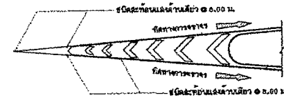
การติดตั้งปูมะทอนแสงที่เส้นคั่นกลางทาง
