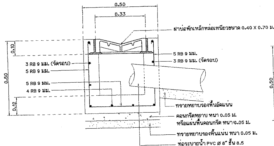
แบบขยายบ่อพักระบายน้ำ คสล. พร้อม ฝาบ่อพักรางวิ
