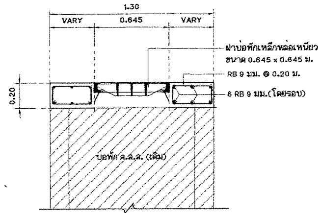
แบบขยายรูปตัด ② การติดตั้งฝาบ่อพักเหล็กหล่อเหนียว 2
