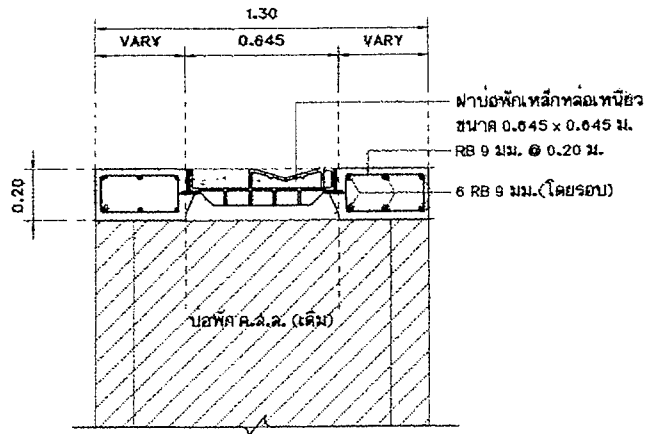
แบบขยายรูปตัด ② การติดตั้งฝาบ่อพักเหล็กหล่อเหนียว 1
