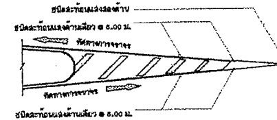
การติดตั้งปูมะทอนแสงเกาะกลางกรณีเดินรถสองทาง
