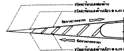
การติดตั้งปูมะทอนแสงที่เส้นแบ่งช่องจราจรและขอบทาง
