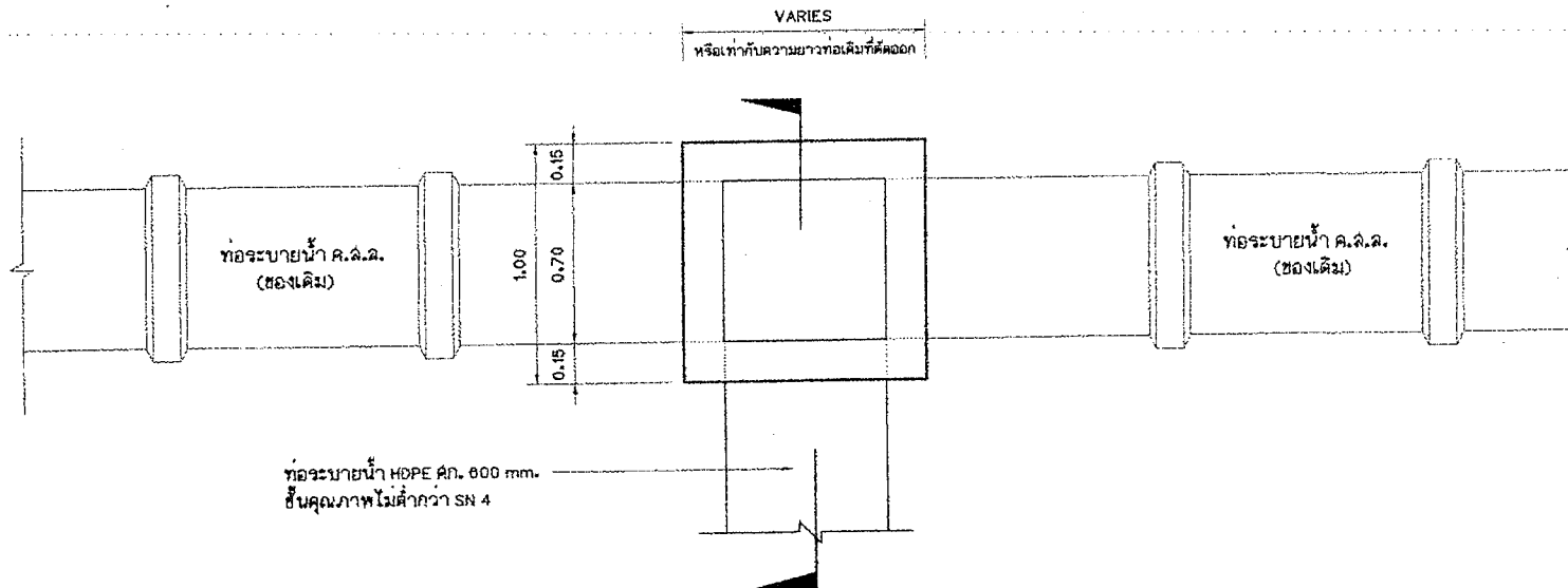
แผนการเชื่อมต่อในกรณีเชื่อมกับท่อระบายน้ำช่องเดิม มาตราส่วน 1:20
