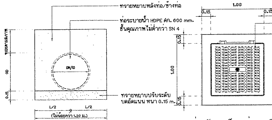
แบบขยายฝาบ่อพักเหล็กหล่อเหนียว 2
