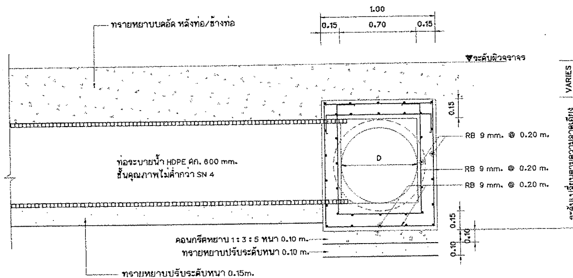
รูปตัดการเชื่อมต่อท่อระบายน้ำช่องเดิม มาตราส่วน 1:20
