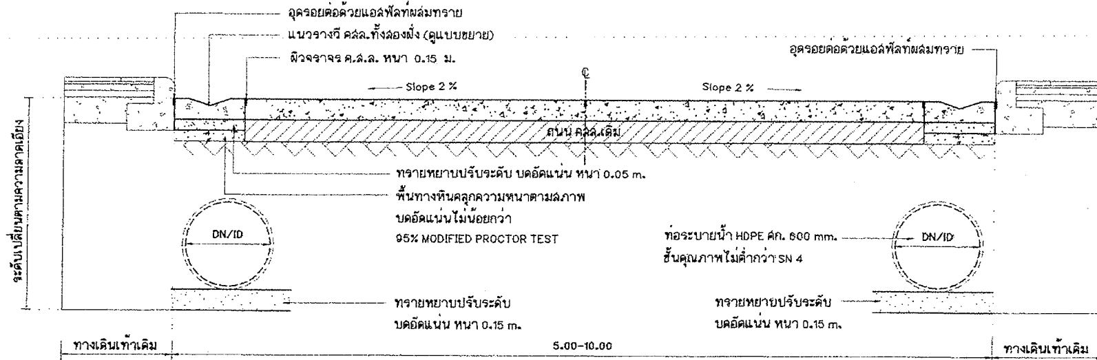
แบบขยายรูปตัด 1
