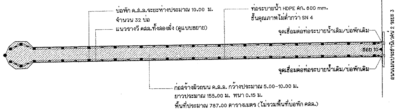
แปลนก่อสร้างปรับปรุงถนน และวางท่อระบายน้ำ มาตราส่วน 1:600
