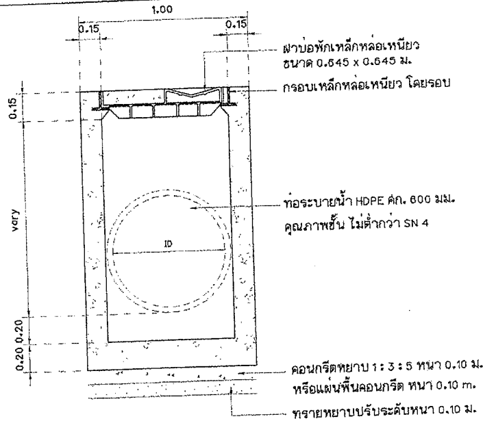
แบบขยายรูปตัด บ่อพัก คลล์.
