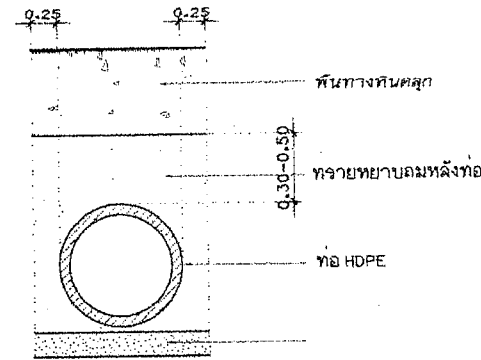
ท่อระบายน้ำ HDPE
