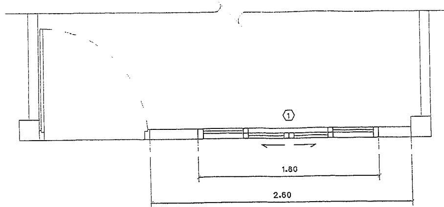
แบบขยาย 3 SCALE 1:25
