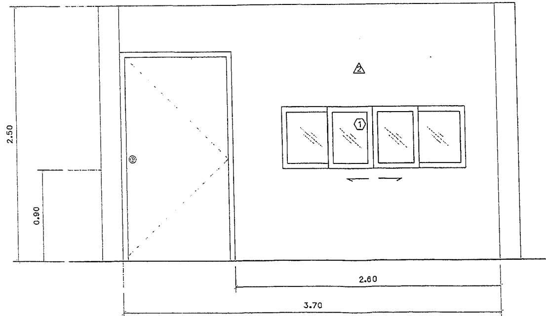
แบบขยาย 3 SCALE 1:25
