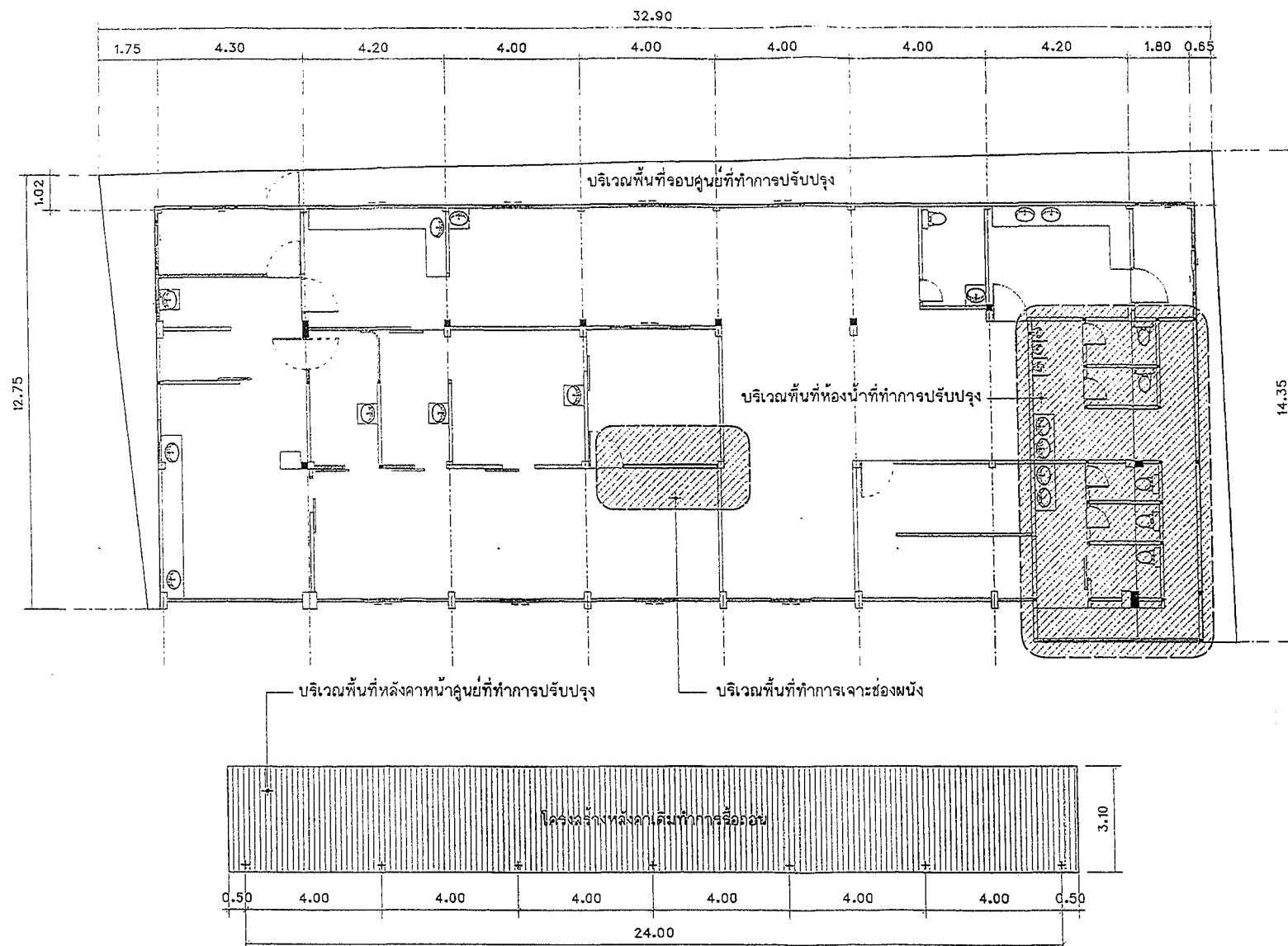
แปลนอาคารศูนย์บริการสาธารณสุข 1 บางพัง (ก่อนปรับปรุง) SCALE 1:125
