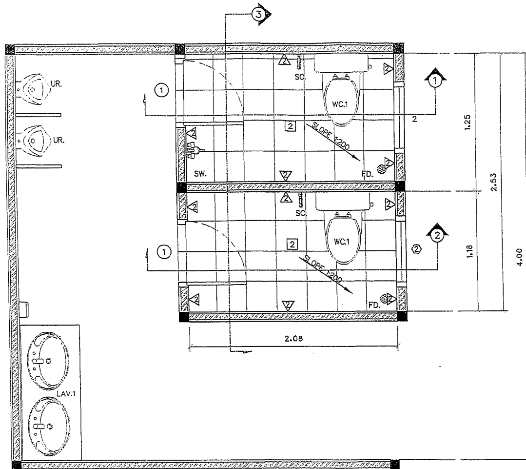
แบบขยาย 2 SCALE 1:50
