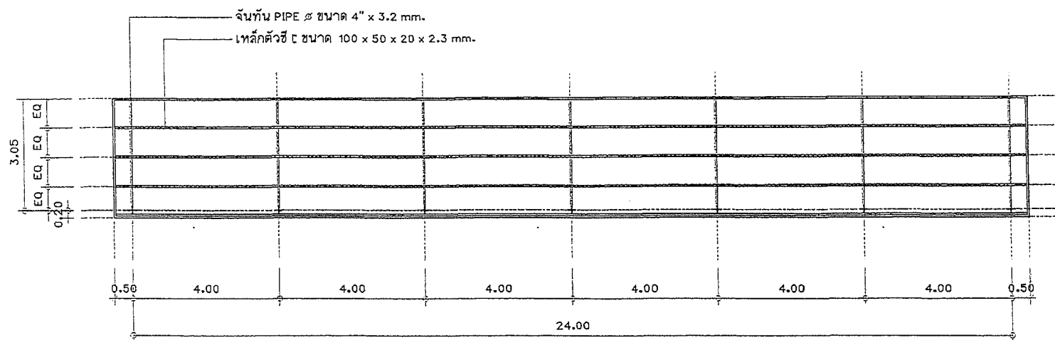
แบบขยาย 5 SCALE 1:100
