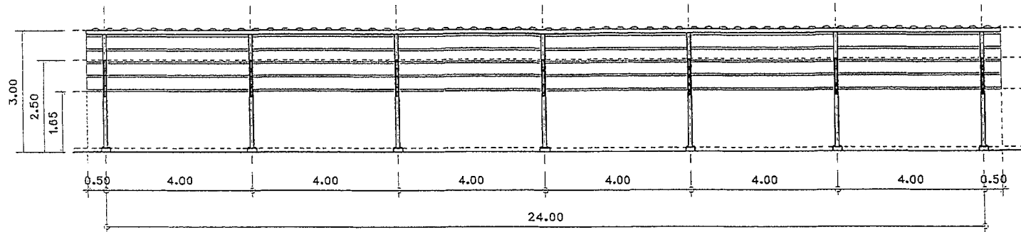
รูปด้าน ① SCALE 1:100
