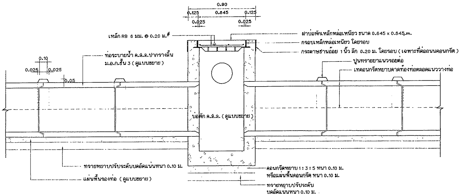
รูปตัดตามยาวของการวางทอระบายน้ำ มาตราส่วน 1:20
