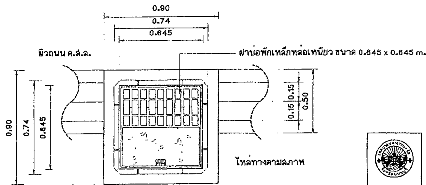
แบบขยายแปลนรางวี
