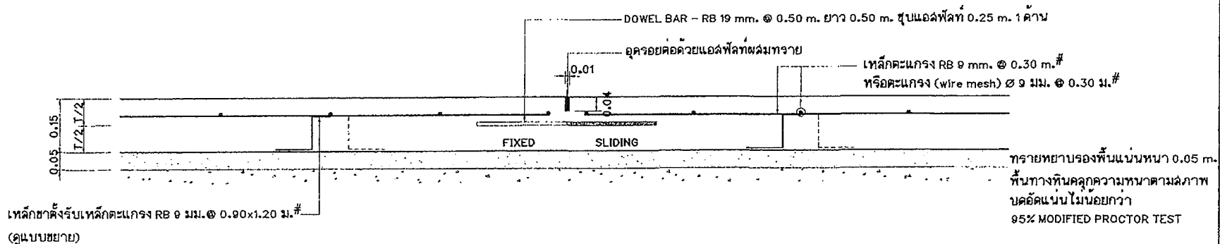
แบบขยาย TRANSVERSE JOINT มาตราส่วน 1:10 ทุกระยะ 6.00 m.
