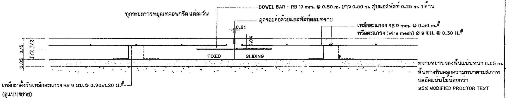
แบบขยาย CONSTRUCTION JOINT มาตราส่วน 1:10
