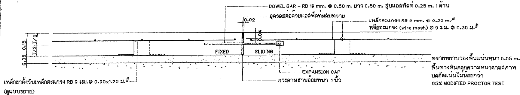
แบบขยาย EXPANSION JOINT มาตราส่วน 1:10 ทุกระยะ 30.00 m.
