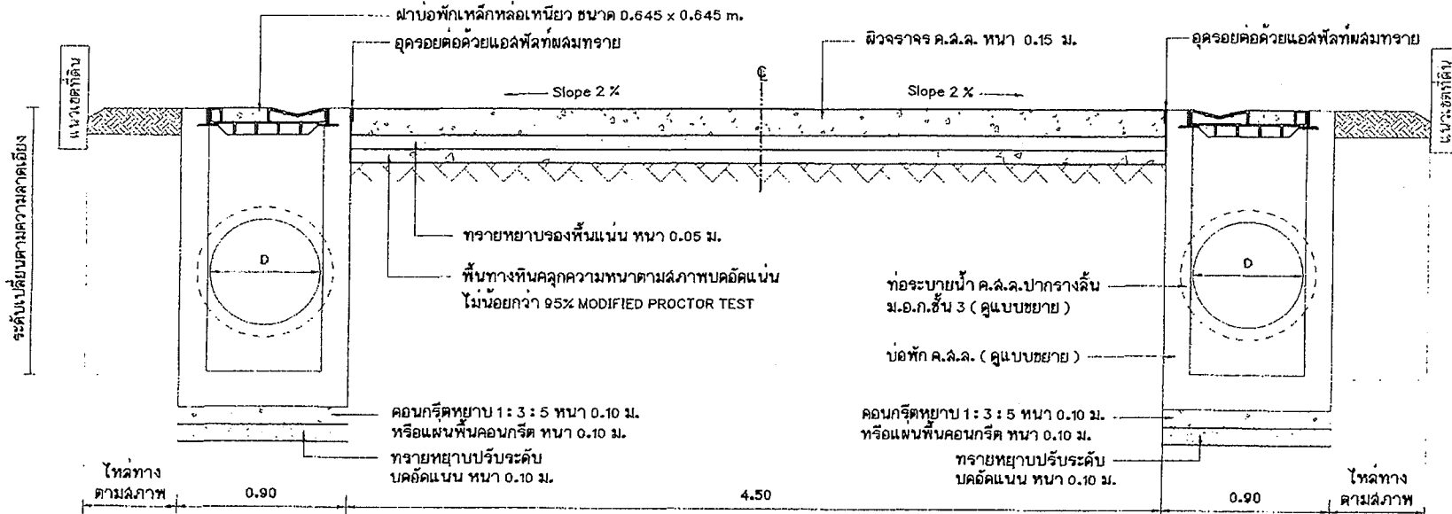
แบบขยายรูปตัด 2 มาตราส่วน 1 : 20
