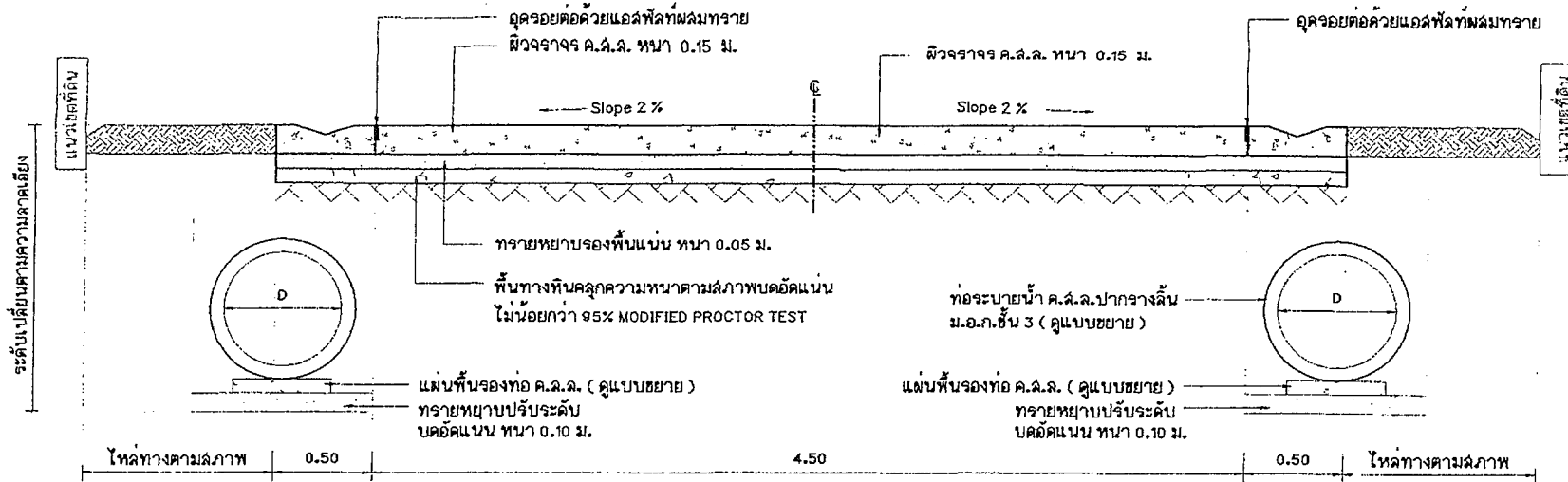
แบบขยายรูปตัด 1 มาตราส่วน 1 : 20
