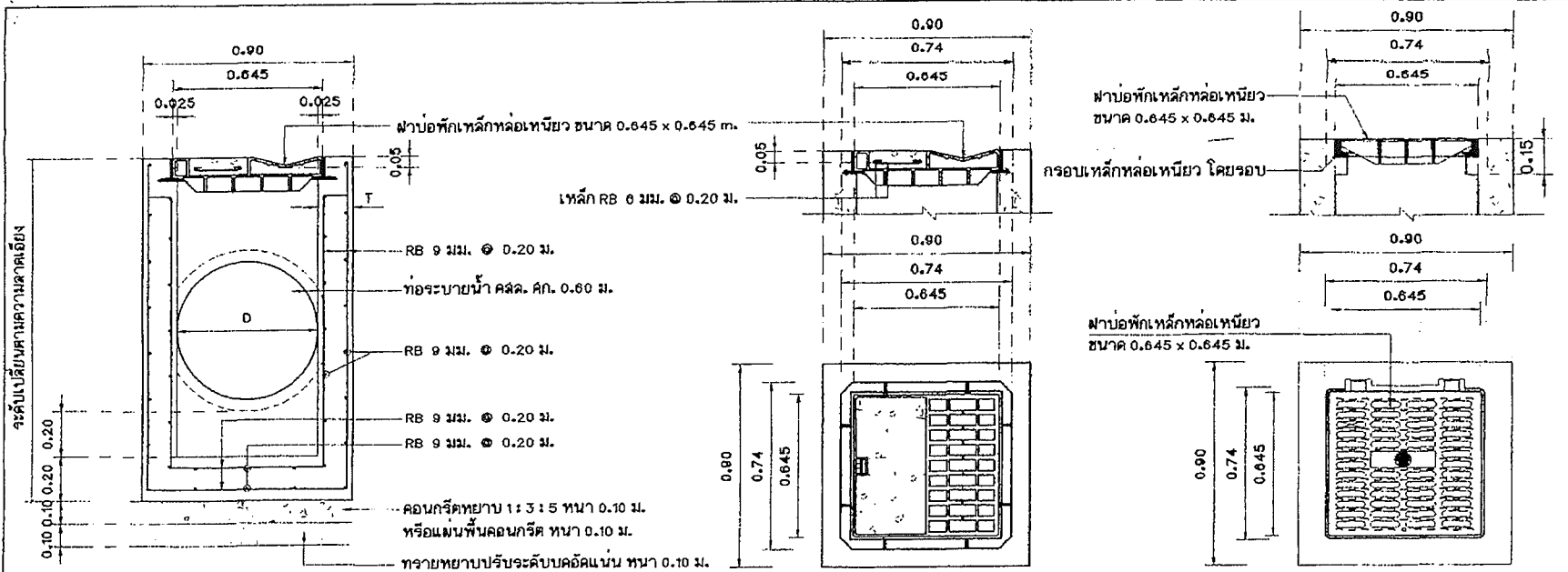
แบบขยายบ่อพัก ค.ล.ล.
