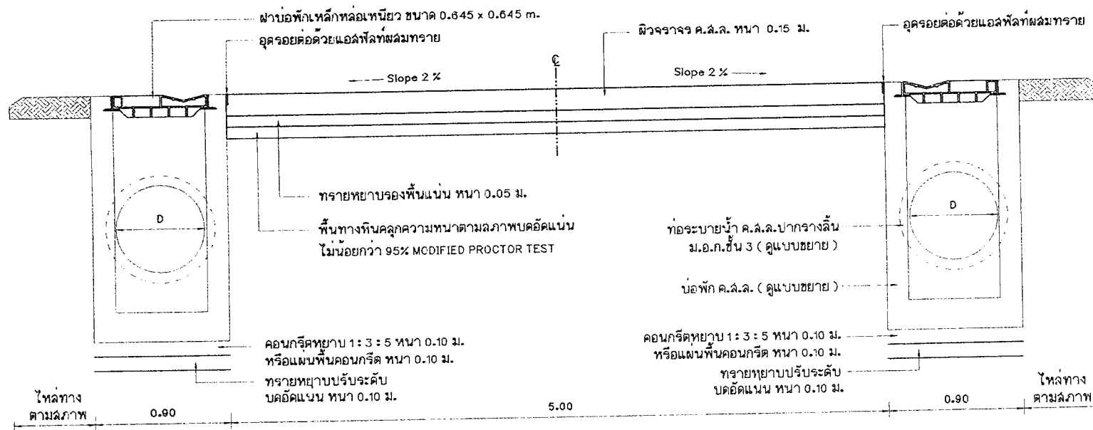
แบบขยายรูปตัด 2 มาตราส่วน 1:20
