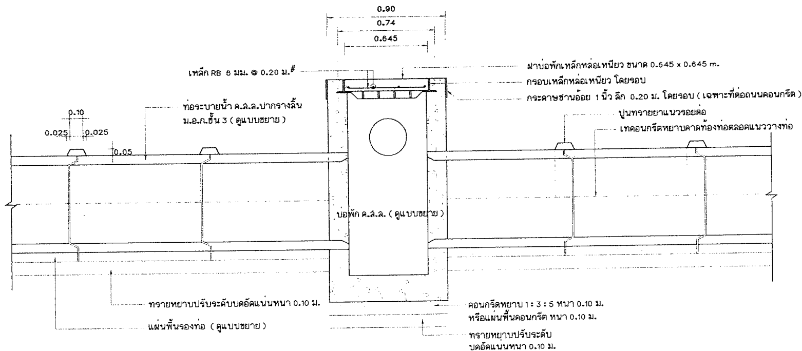
รูปตัดตามยาวการวางท่อระบายน้ำ ปู มาตราส่วน 1:20
