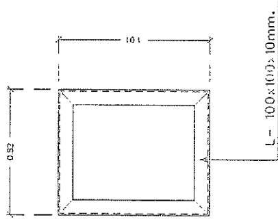
แบบขยาย 1 ขนาดฐาน 1 : 25
