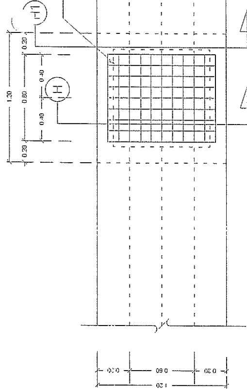
แบบขยายวงรับน้ำหนัก (MH3)
