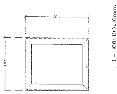
แบบขยาย 2
