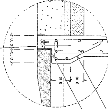
เหล็กฉากกรัดรอบฝาปิด เหล็ก L-100x100x10 มม.
