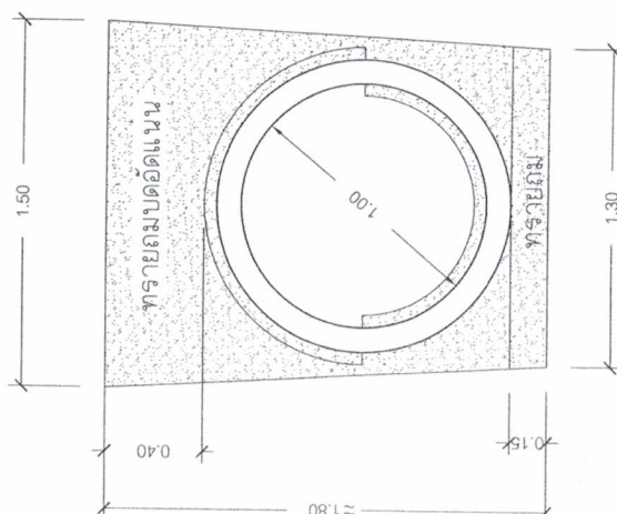
รูปตัด I ทอระบายน้ำ ค.ส.ล. ปาตราชลวน 125
