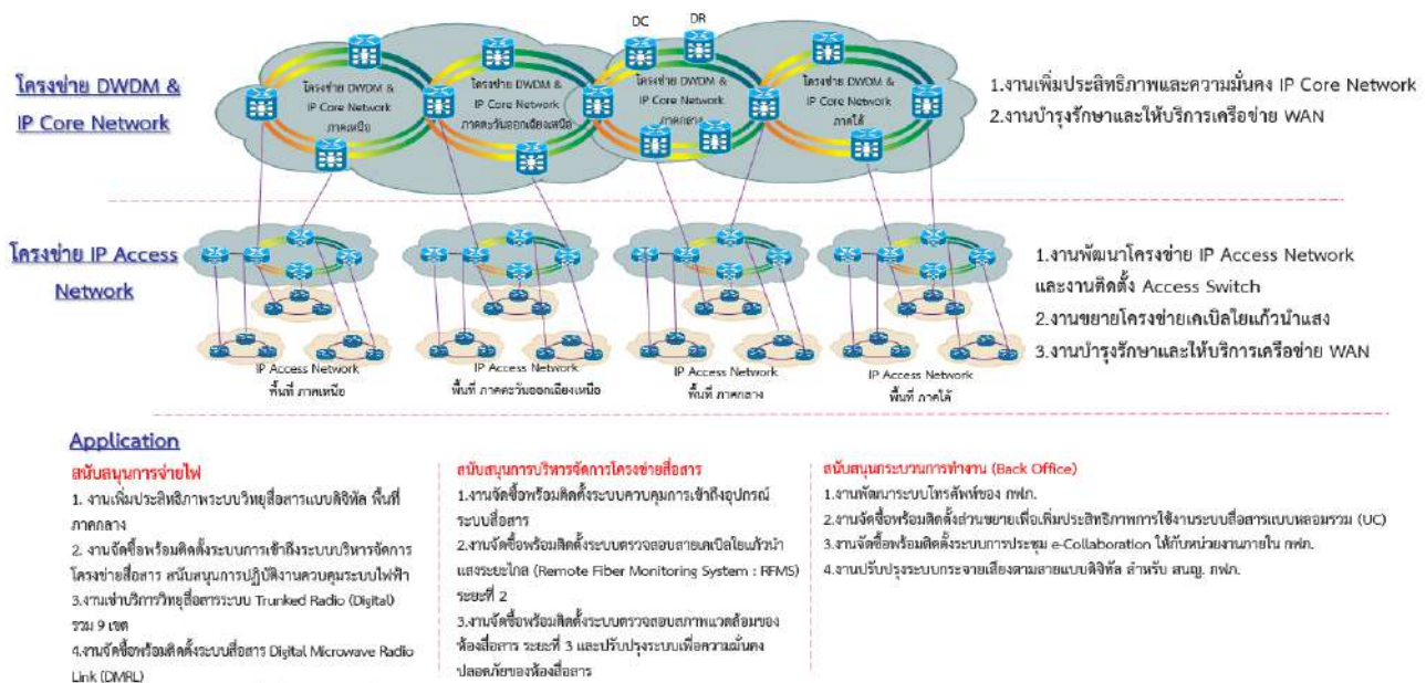
รูปที่ 14-10 ภาพรวมโครงสร้างพื้นฐานด้านการสื่อสารของ กฟภ.
