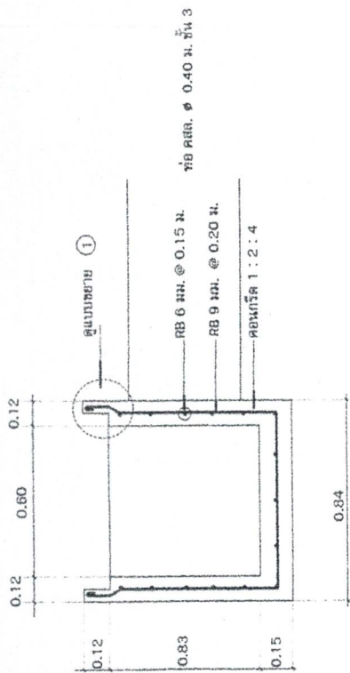
รูปตัด ก - ก
