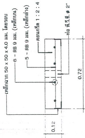
รูปตัดฝายปิดบ่อพัก
