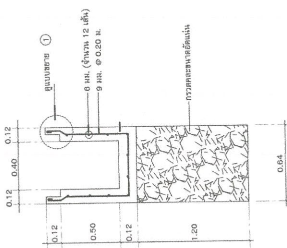
รูปตัดขวางระบบซึม
