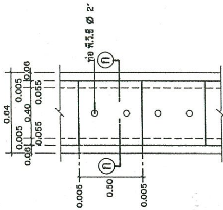
แปลนร่างระบายน้ำ คสล. รูปตัวยู
