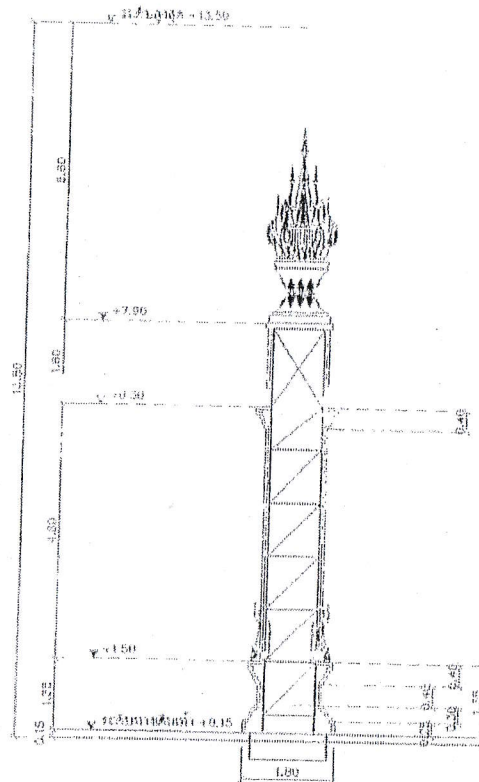
รูปด้านข้าง หน้าบ้าน 1 : 25
