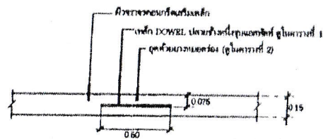
CONTRACTION JOINT ทุกระยะไม่เกิน 10.00 ม. มาตราส่วน NOT TO SCALE
