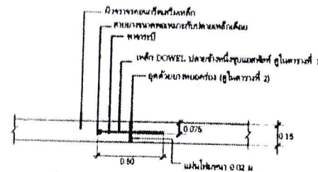
EXPANSION JOINT ทุกระยะไม่เกิน 100.00 ม. มาตราส่วน NOT TO SCALE
