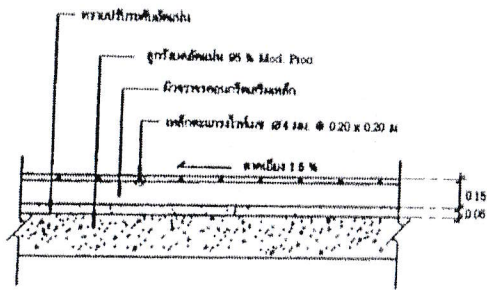
รายละเอียดถนนคอนกรีตเสริมเหล็ก มาตราส่วน NOT TO SCALE
