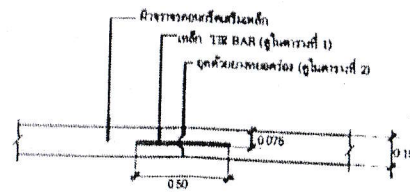
LONGITUDINAL JOINT มาตราส่วน NOT TO SCALE
