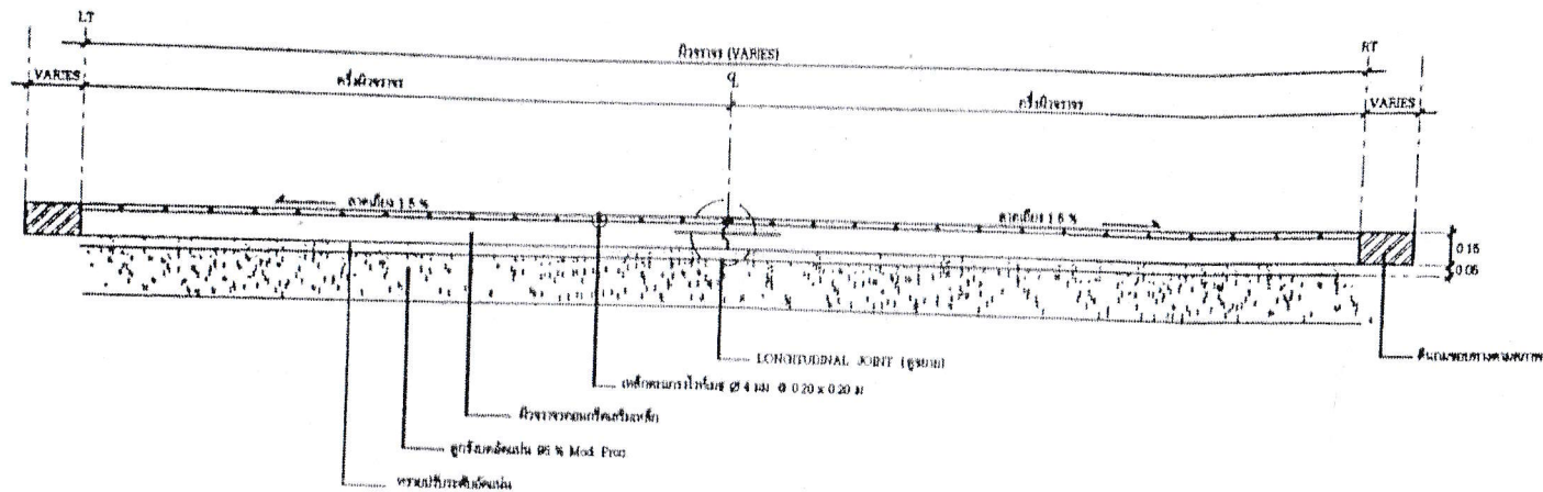
รูปตัดตามขวางผิวจราจร มาตราส่วน NOT TO SCALE
