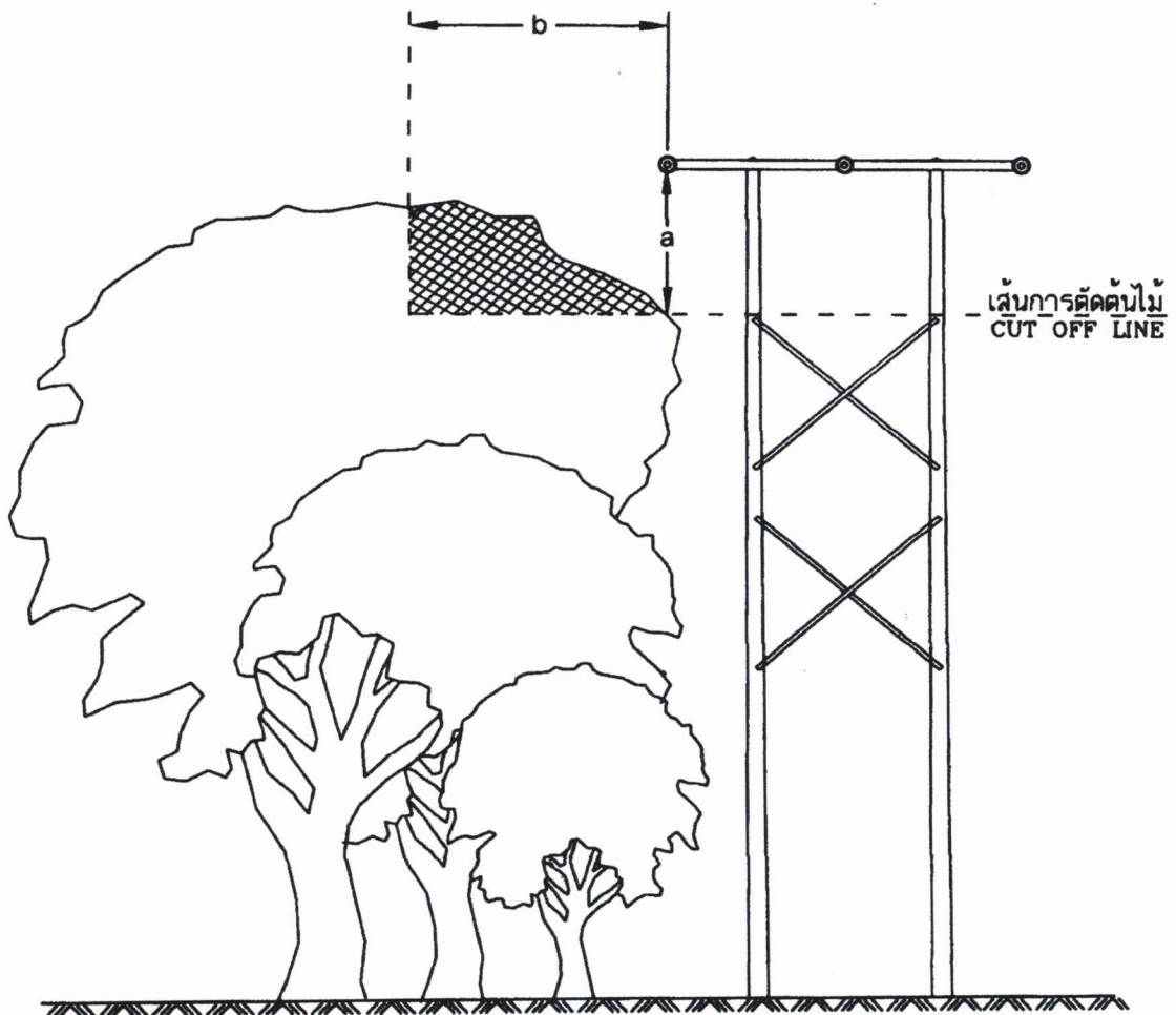
การตัดแต่งต้นไม้สำหรับสายเบสเปลือยแรงสูงที่มีระยะห่างระหว่างเสาดั้งแต่ 100 เมตร ขึ้นไป TREE TRIMMING FOR H.V. BARE CONDUCTOR WITH SPANS OF 100 m AND ABOVE.
