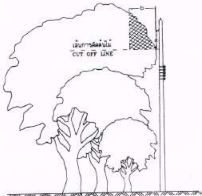
การตัดแต่งต้นไม้สำหรับสายหุ้มฉนวนเต็มพิกัดบิดเกลียว TREE TRIMMING FOR TWISTED AERIAL CABLE.
