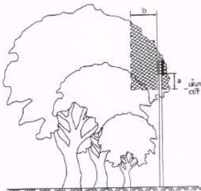
การตัดแต่งต้นไม้สำหรับสายหุ้มฉนวนแรงต่ำ หรือสายพันรวม หลายแกน หรือสายคิ๊ปโถงบน TREE TRIMMING FOR L.V. INSULATED OR MULTIPLEX CABLE OR STREET LIGHTING CABLE.
