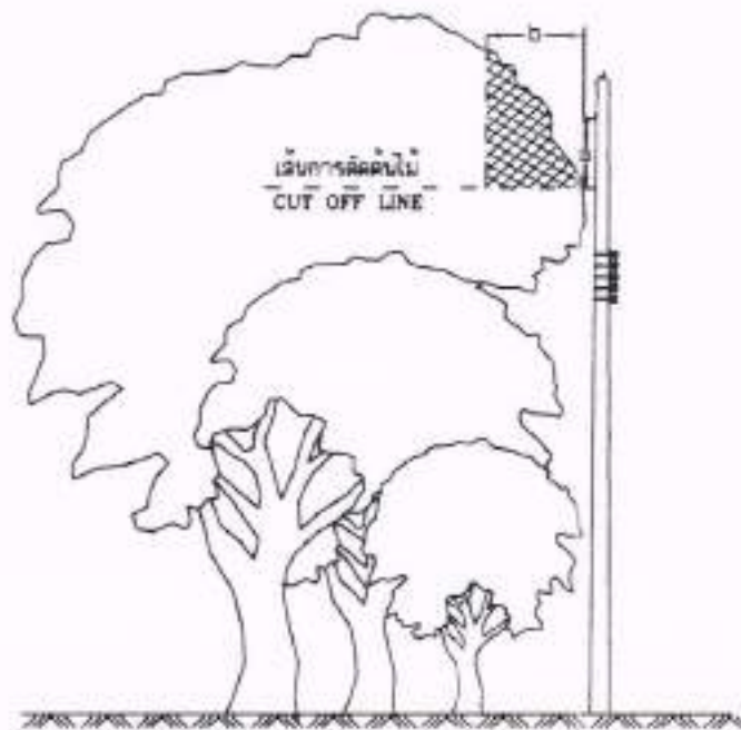
การตัดแต่งต้นไม้สำหรับสายหุ้มฉนวนเต็มพิกัดดัดโค้ง TREE TRIMMING FOR TWISTED AERIAL CABLE.
