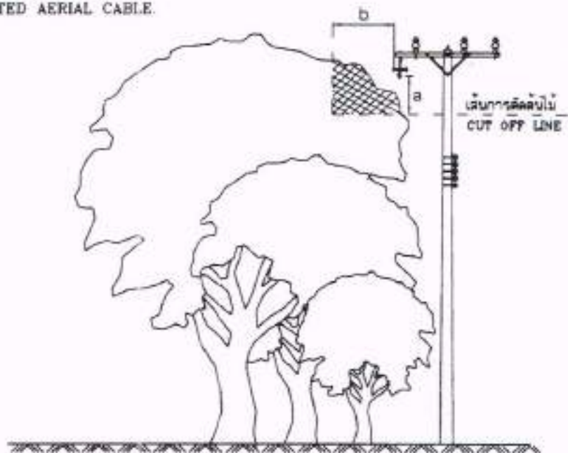
การตัดแต่งต้นไม้สำหรับสายหุ้มฉนวนแบบไม่เต็มพิกัดหรือดัดเบิดอากาศ TREE TRIMMING FOR PARTIALLY INSULATED CONDUCTOR OR SPACED AERIAL CABLE.
