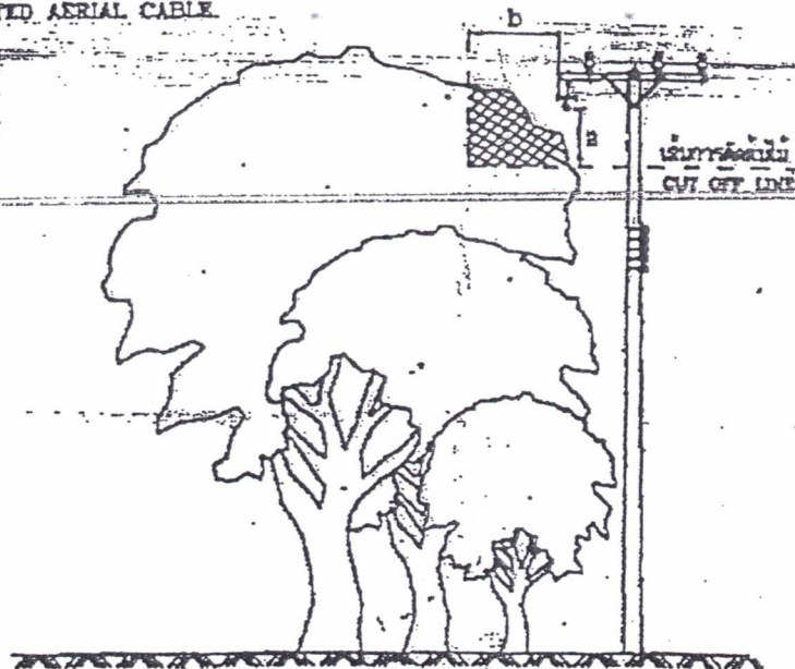
การตัดแต่งต้นไม้สำหรับสายหุ้มฉนวนแบบไม่เต็มทึดหรือสายเปลือยอากาศ TREE TRIMMING FOR PARTIALLY INSULATED CONDUCTOR OR SPACED AERIAL CABLE
