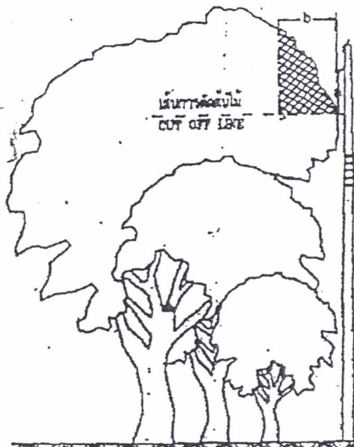
การตัดแต่งต้นไม้สำหรับสายหุ้มฉนวนแบบบิดเกลียว TREE TRIMMING FOR TWISTED AERIAL CABLE
