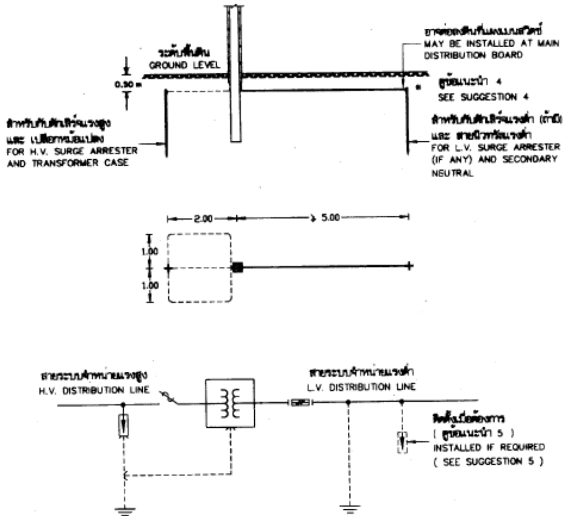
ไดอะแกรมแสดงการต่อลงดิน EARTHING DIAGM
