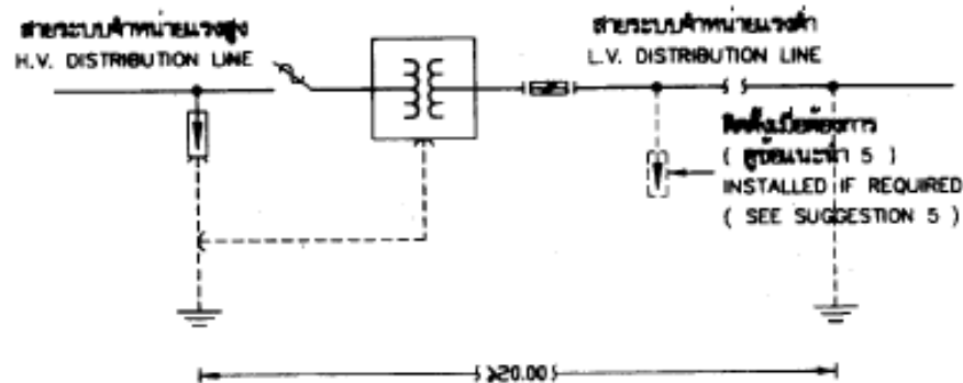
ไดอะแกรมแสดงการต่อดิน EARTHING DIAGRAM
