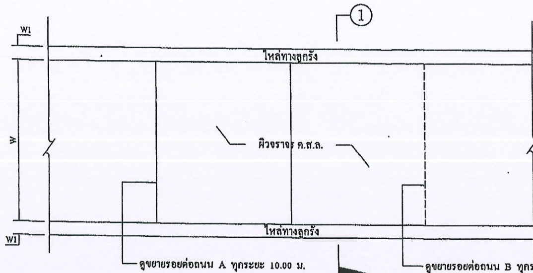
แปลนถนน ค.ส.ล.
