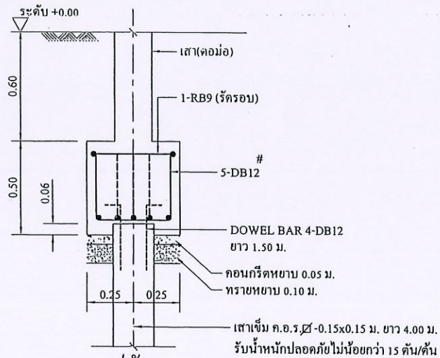
รูปตัด 1 มาตราส่วน 1:25
