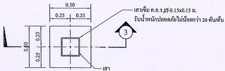
แปลนฐานราก F1 มาตราส่วน 1:25
