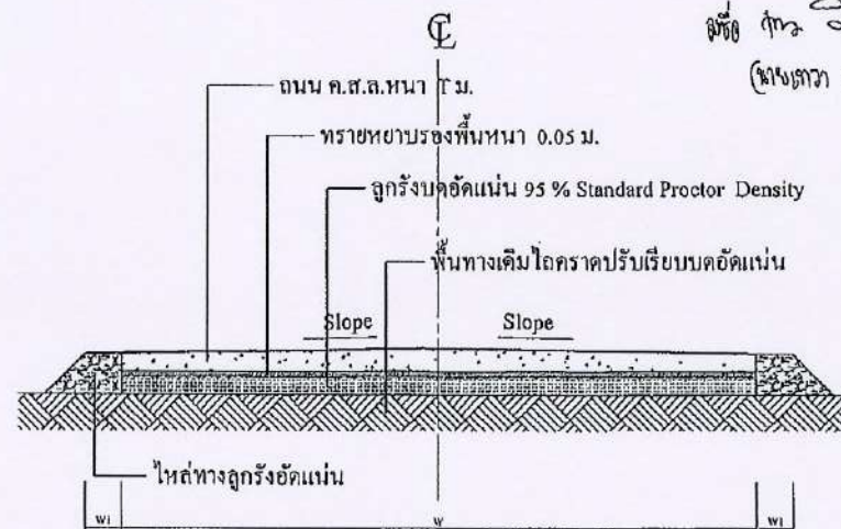
รูปตัด I
