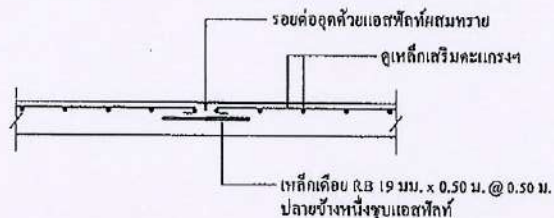
ขยายรอยต่อถนน A (ทุกระยะ 10.00 ม.)
