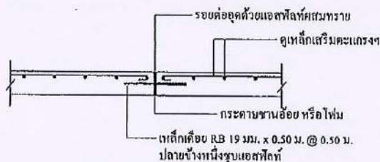
ขยายรอยต่อถนน B (ทุกระยะ 50.00 ม.)
