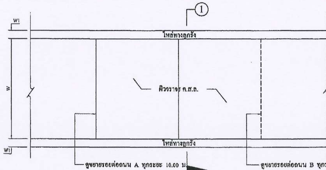
แปลนถนน ค.ส.ล.
