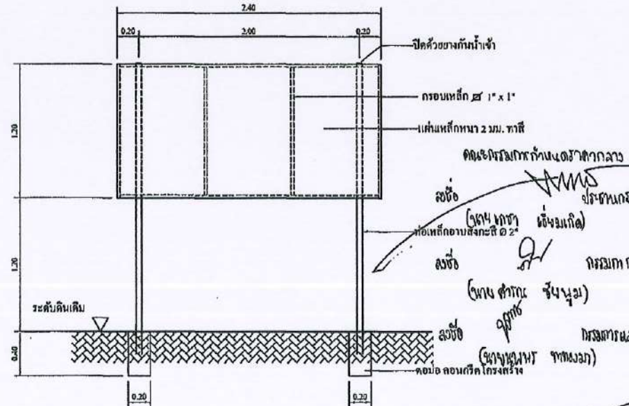
แสดงรายละเอียดโครงสร้างป้าย
