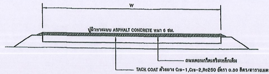
รูปตัดตามขวางโครงสร้างทาง not to scale
