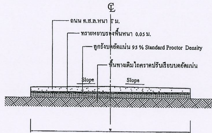
รูปตัด 1
